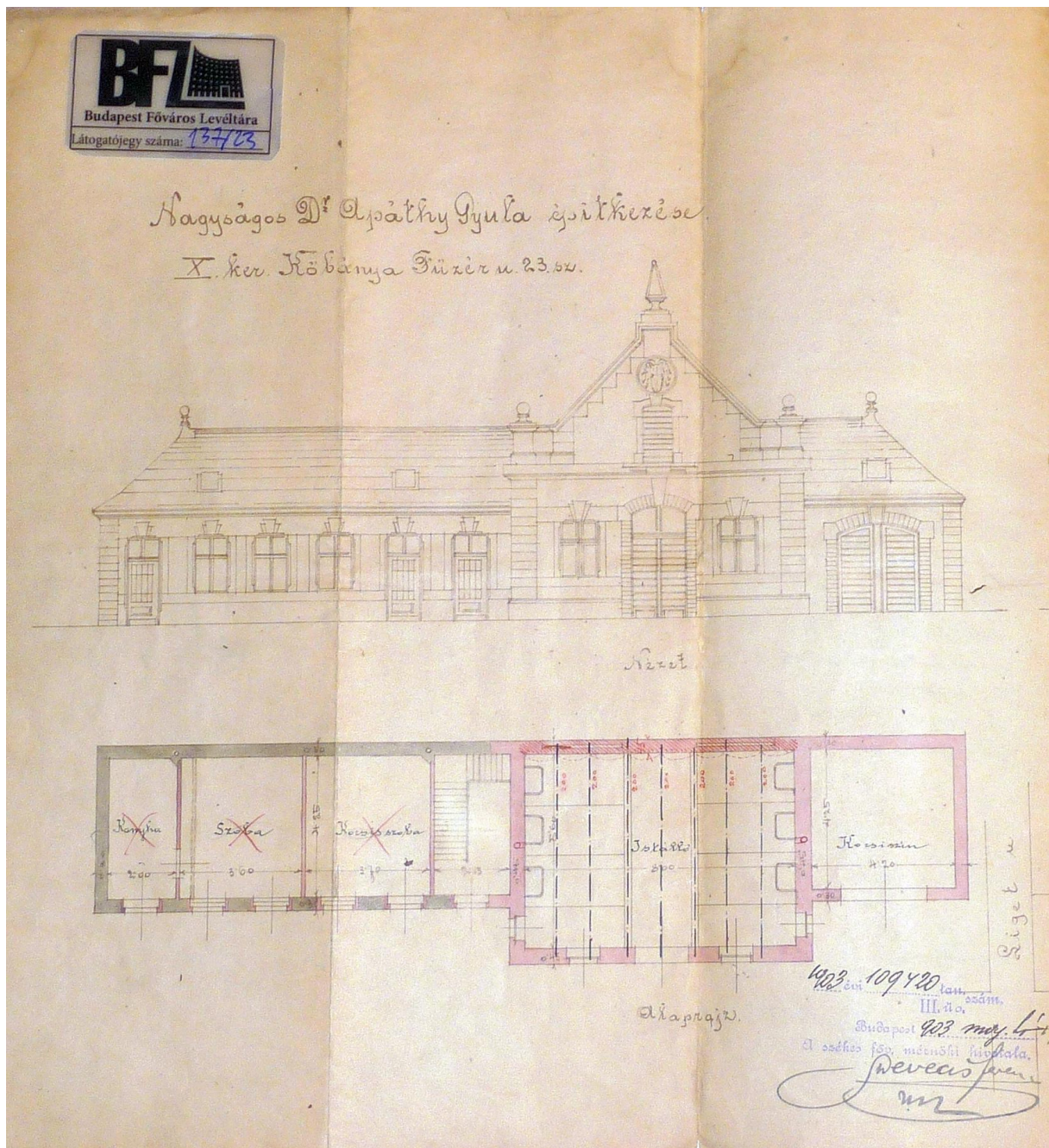
16. kép: Részlet a HU.BFL XV.17.d.329.39051/1 jelzetű tervlapról (13. kép) Melléképület alaprajz, nézet - 1903
