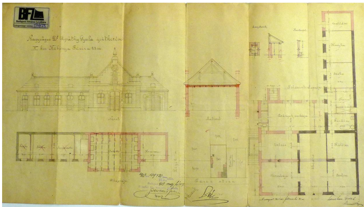
13. kép: HU.BFL XV.17.d.329.39051/1 - Landherr Gyula és Devecsis Ferenc terve – 1903 Nagyságos Dr. Apáthy Gyula építkezése X. ker. Kőbánya Füzér u. 23.
