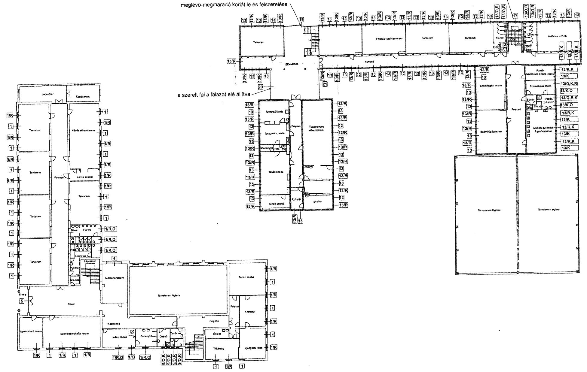
TERVEZETT I.EMELETI ALAPRAJZ
