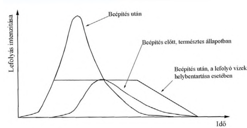
23. ábra: A beépítés hatása a felszíni lefolyásra (Wright-Heaney, 2001)
