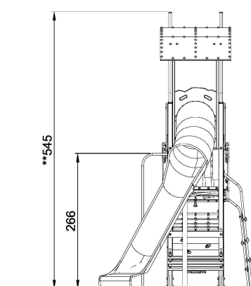
NAT520 1:100
