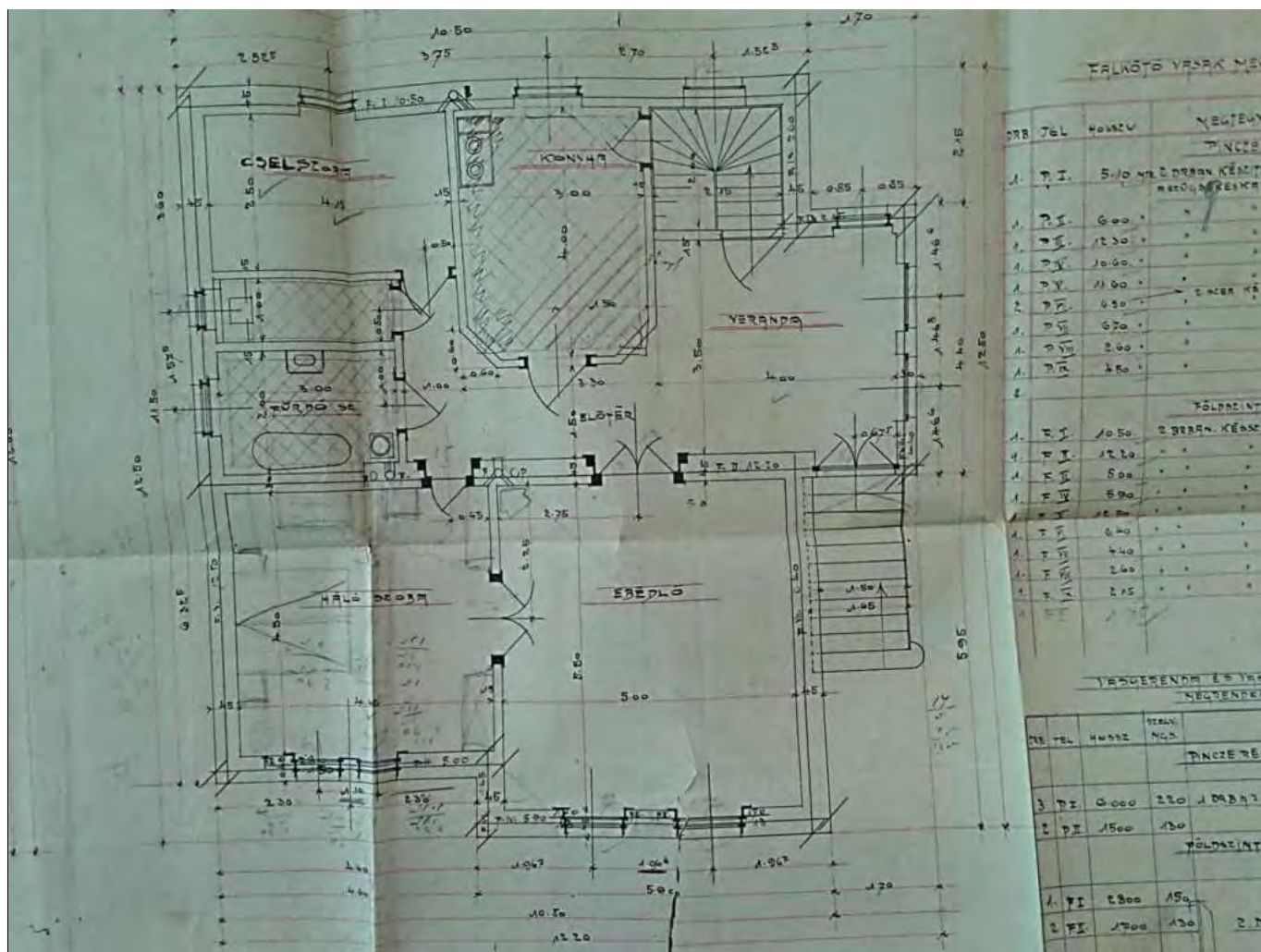
Kiviteli terv a Sorg hagyatékban
