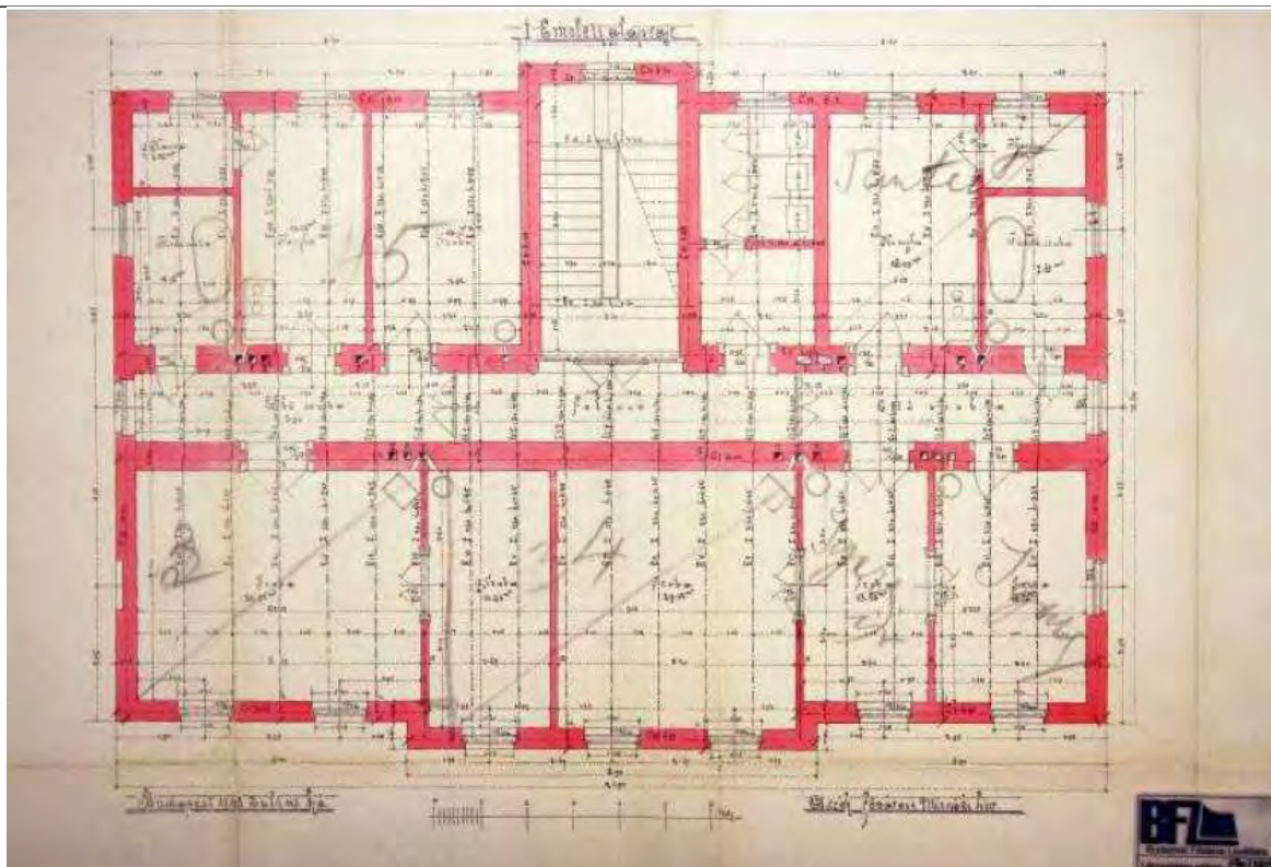
Emeleti alaprajz
