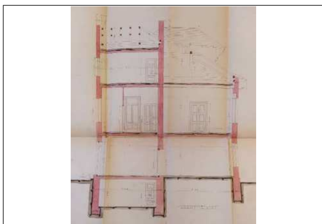
Laboratórium épület terve – metszet (1906)
