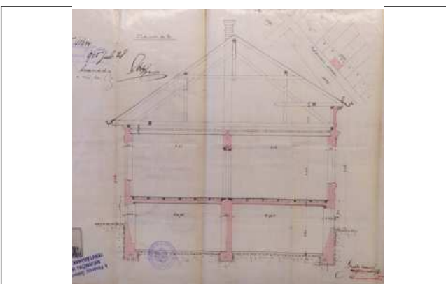
Metszet
