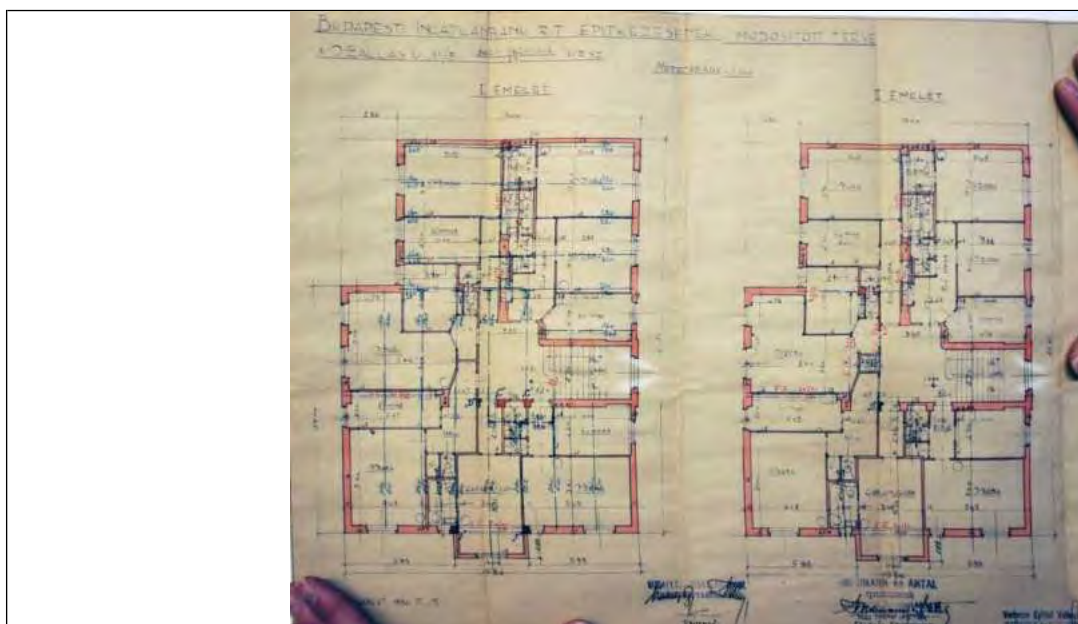
Első és második emelet alaprajza
