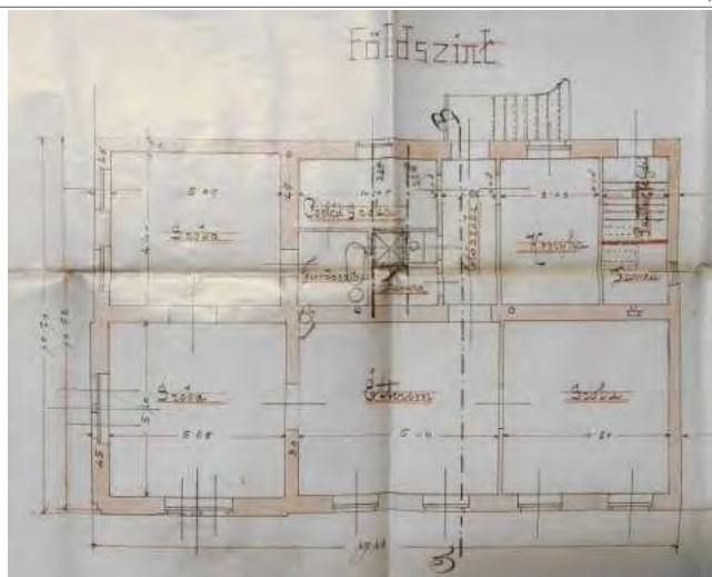
Alaprajzok: földszint és pince
