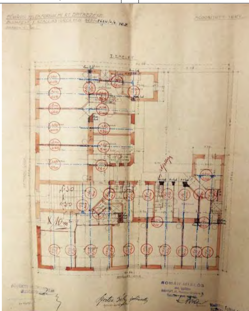
Első emelet alaprajza
