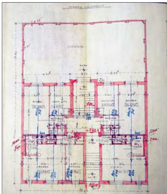
Földszinti alaprajz
