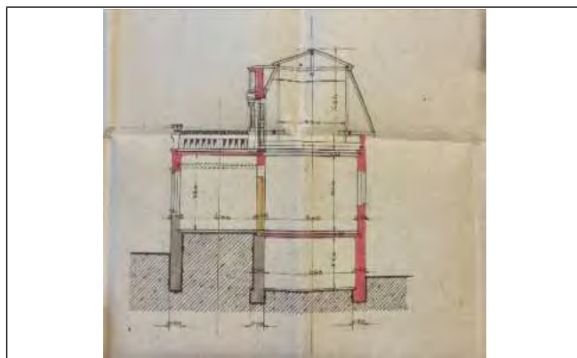
Metszet
