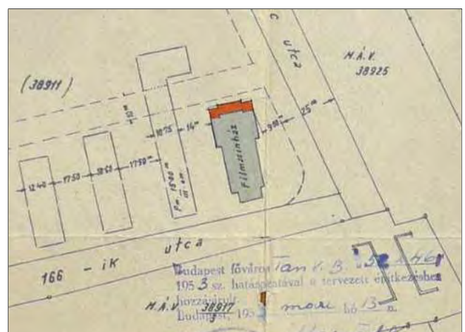
Az egykori moziépület 1952-53-as bővítési terve: a telep déli főtengelye menti előtere megszűnt az épület 5,2 m-es meghosszabbításával
