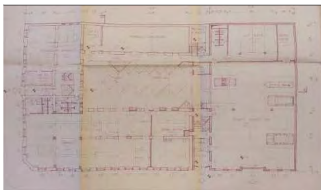
Földszinti alaprajz – Várhivatal rekonstrukció (1986)
