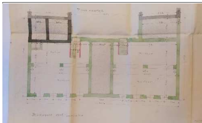
Pincszinti alaprajz (módosított terv, 1935.)
