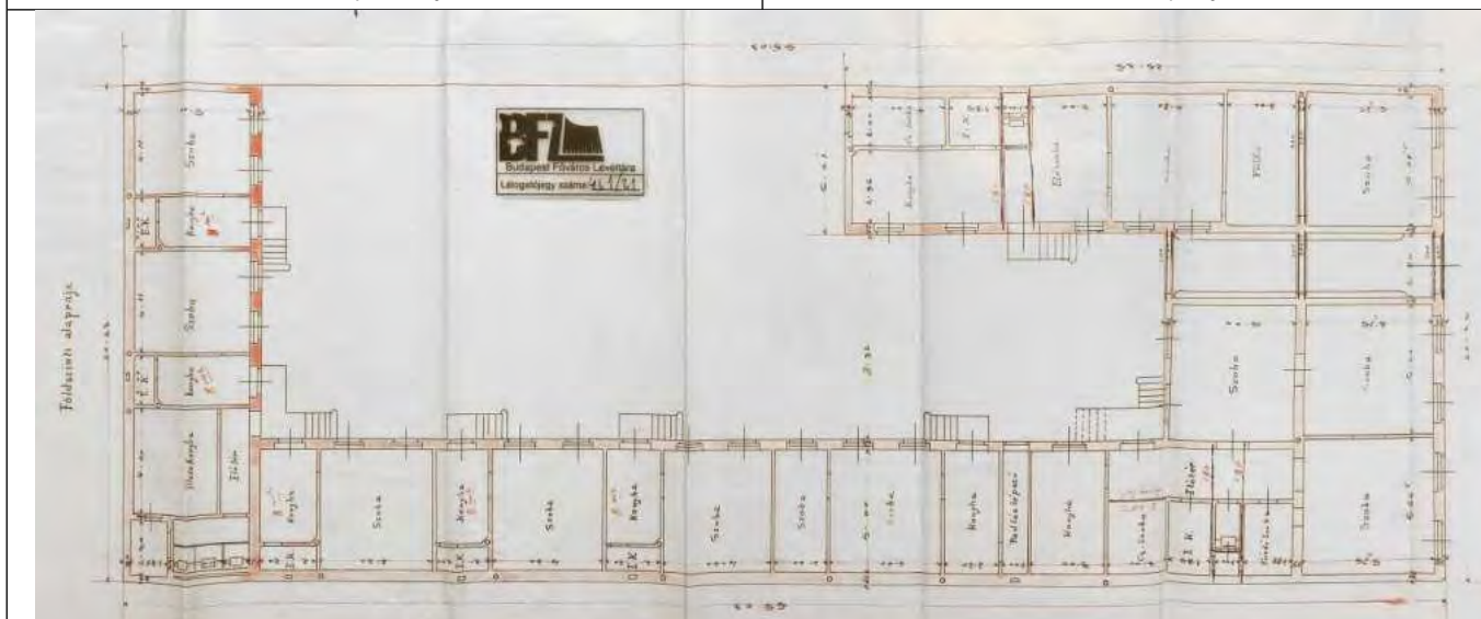
Földszint alaprajz
