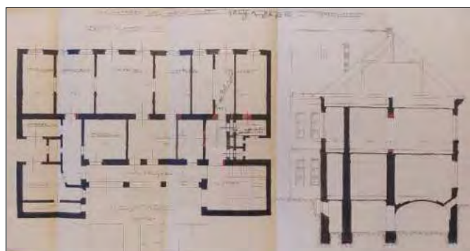
1911-es átalakítási terv
