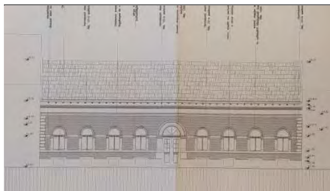
Homlokzaffelújítás terve (2000)
