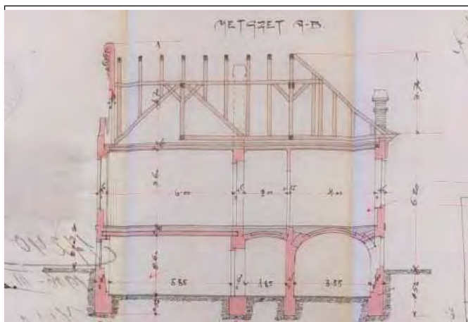
Metszet
