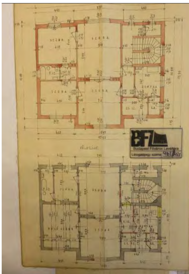
Alaprajzok: felül az emeletráépítés alaprajza
