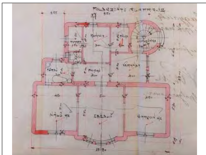
Földszinti alaprajz
