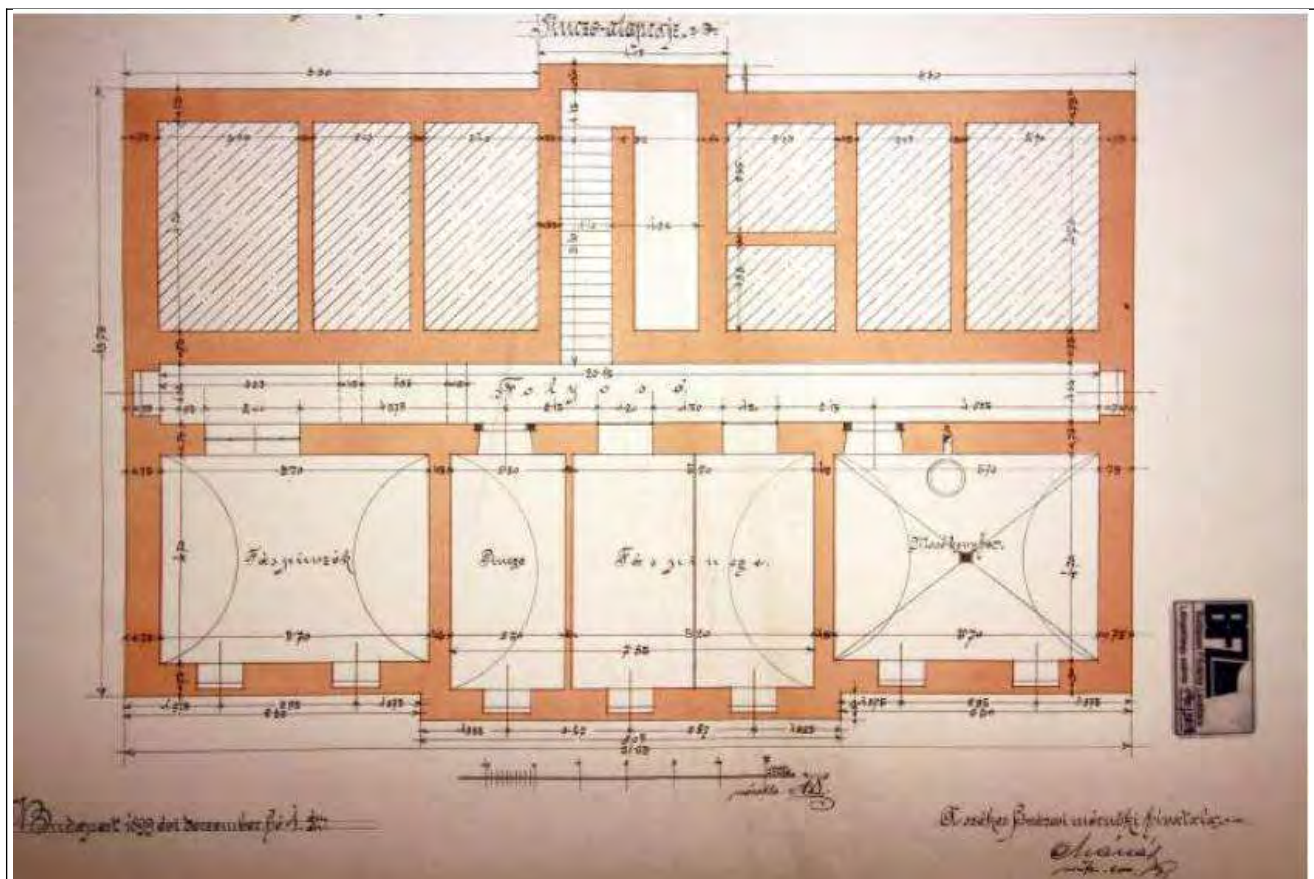
Pince alaprajz
