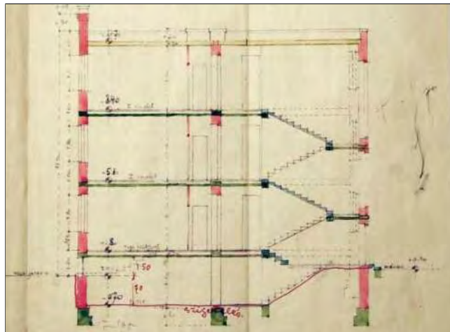
Metszet
