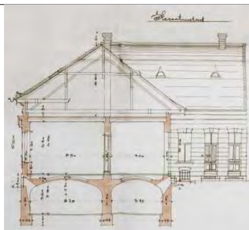
Metszet 1898.
