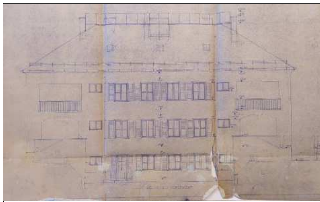
DK-i homlokzat
