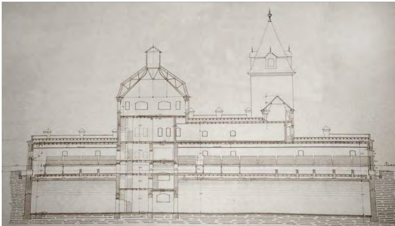
Az eredeti terv részlete 1909-ből (forrás: Sörgyár)
