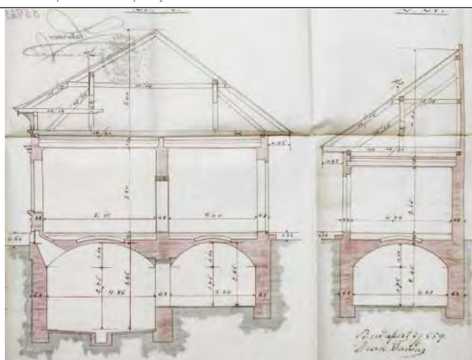
Homlokzat és metszet
