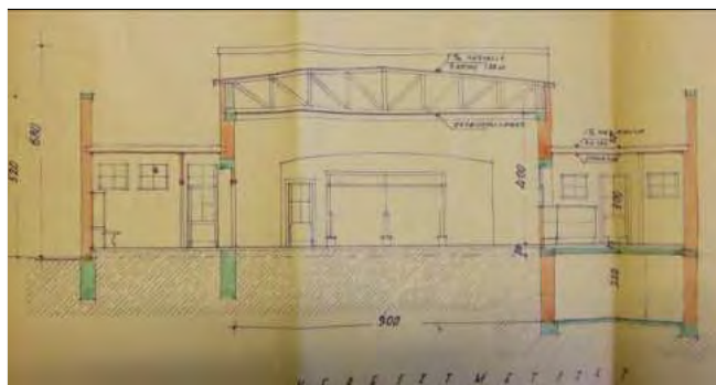
Metszet 1.
