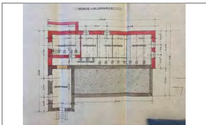
Pince alaprajz
