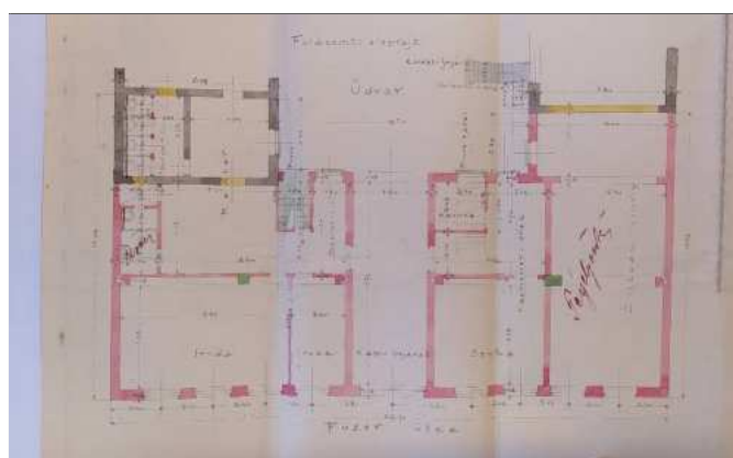
Földszinti alaprajz (módosított terv, 1935.)
