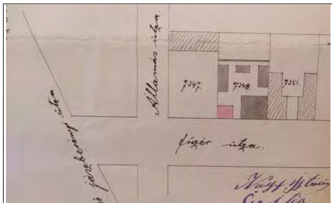
1879-es helyszínrajz
