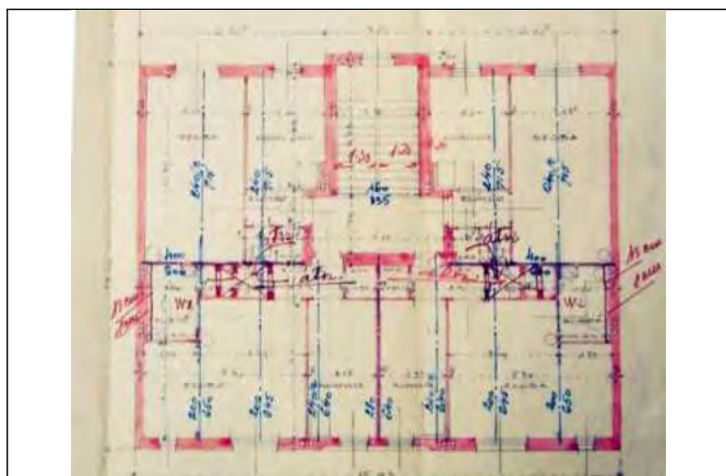
Első emelet alaprajz
