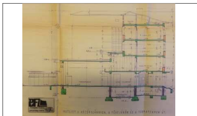
Metszet
