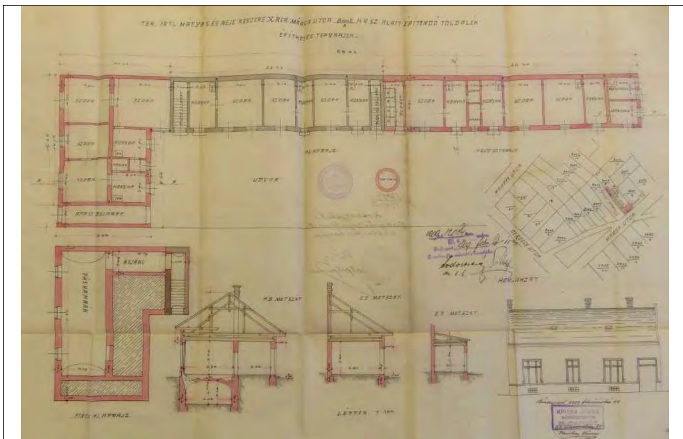
Lakóház tervei
