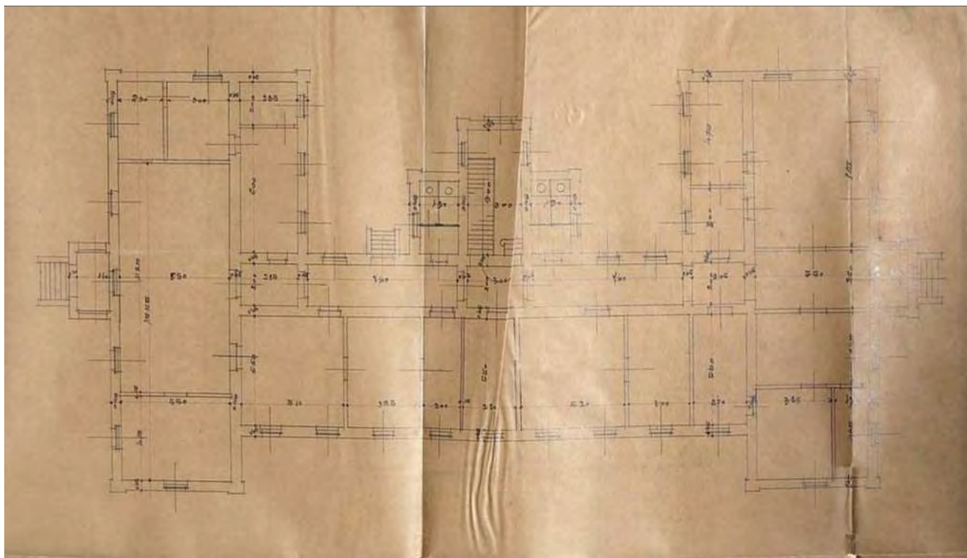
Az épület földszinti alaprajza, évszám és a tervező megnevezése nélküli tervrajz (forrás: BFL)
