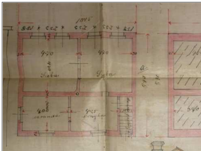
Földszinti alaprajz
