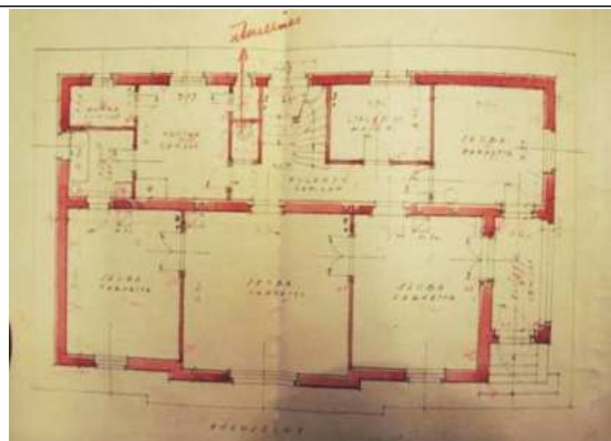
Fabódé terve, 1926. március 13.
