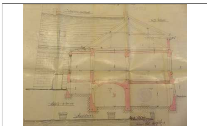
Metszet
