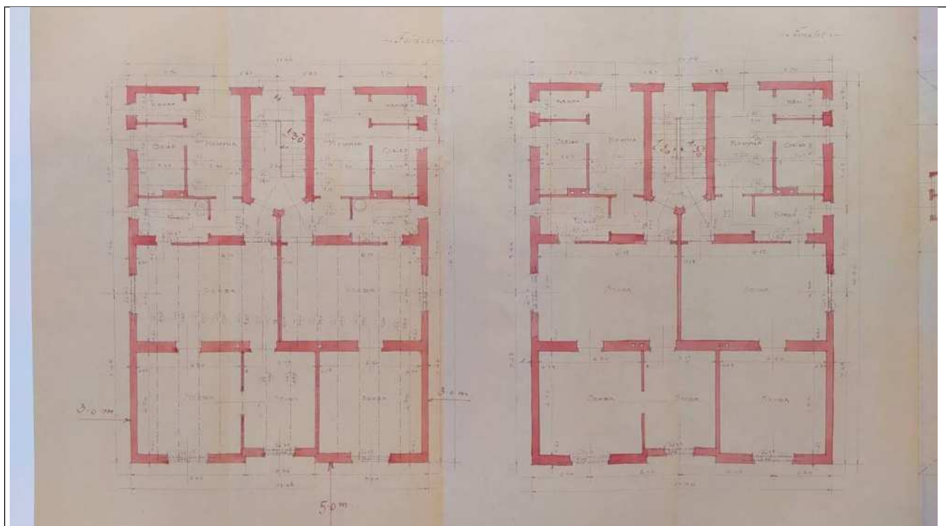
Az utca felőli épületrész földszinti és emeleti alaprajza
