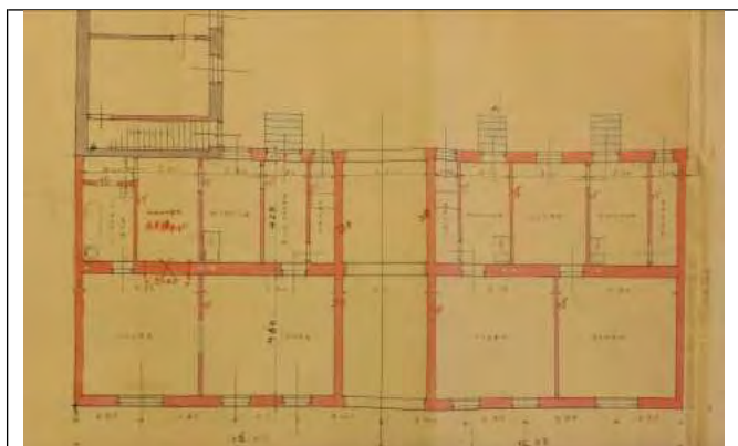
Utcai szárny földszinti alaprajza
