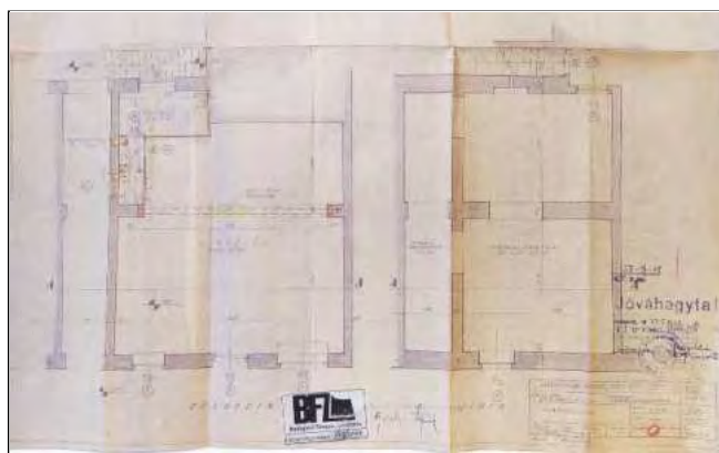
Földszinti és pincszinti alaprajz (1955)
