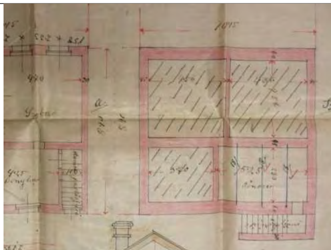
Pince alaprajz
