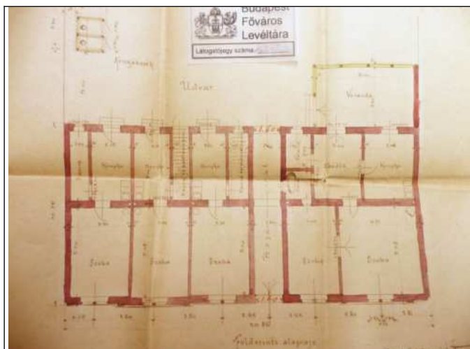
Pince alaprajz
