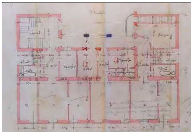
1894-es bérház terve – emeleti alaprajz
