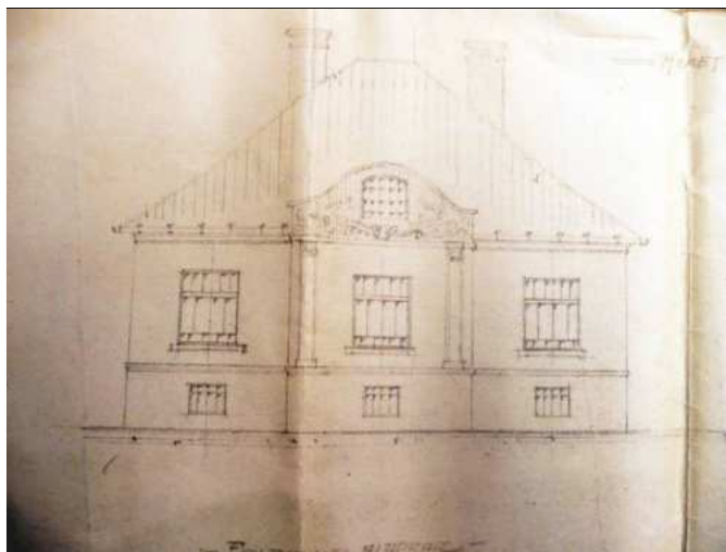
Homlokzat
