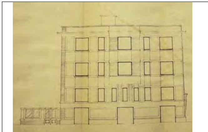
Szállás utcai homlokzat rajza
