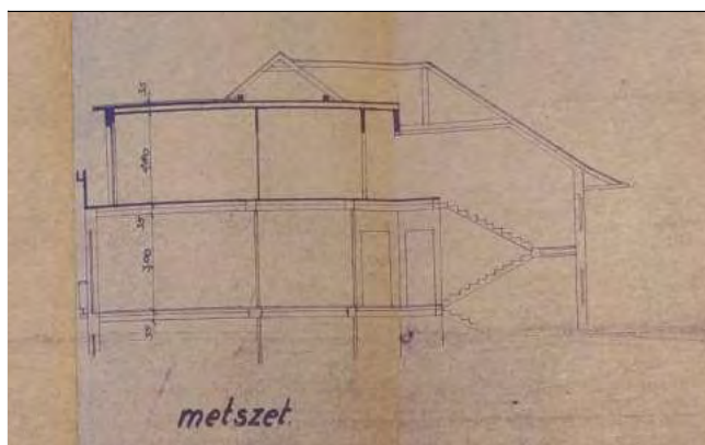
Tetőemeletráépítés tervének metszete (1956)
