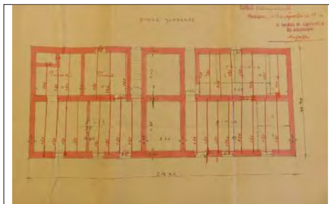
Utcai szárny pincszinti alaprajza
