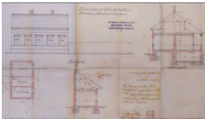
1884-es lakóház terv
