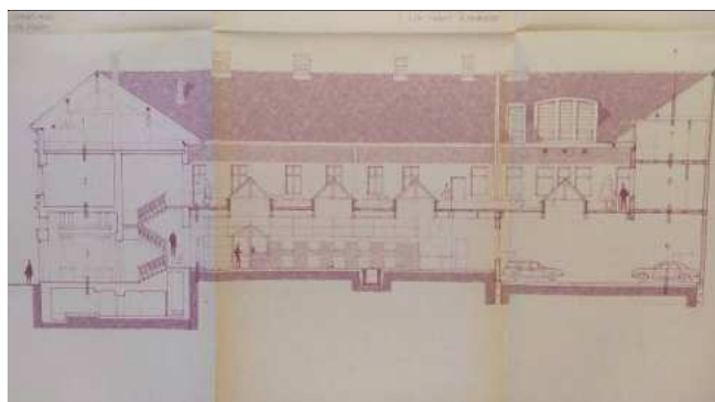
Metszet – Várhivatal rekonstrukció (1986)
