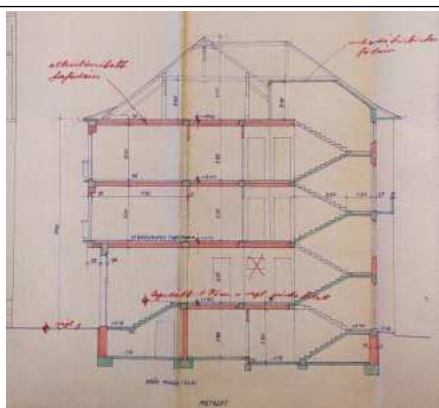
Metszet a tetőemelet ráépítés előtt (1942)
