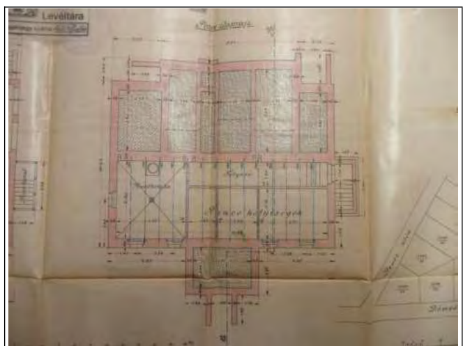
Pince alaprajz
