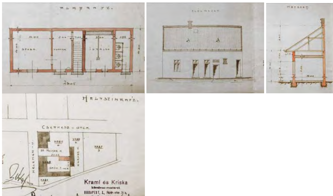
Hátsó épület alaprajza, homlokzata és metszete 1911.
