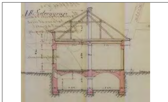
Metszet
