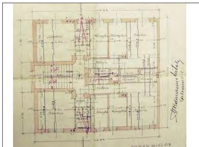
Második emelet alaprajz
