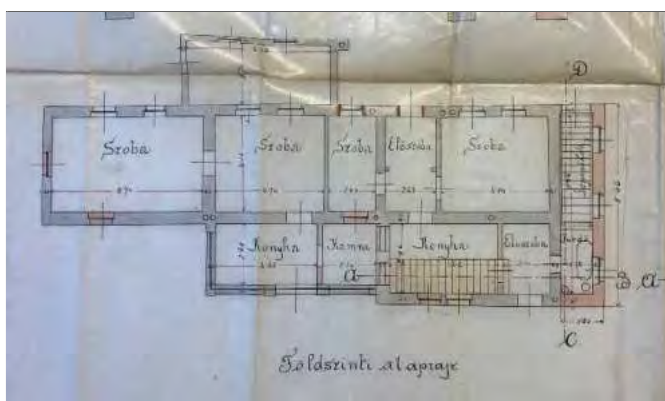
Földszinti alaprajz (toldalékterv, 1899)
