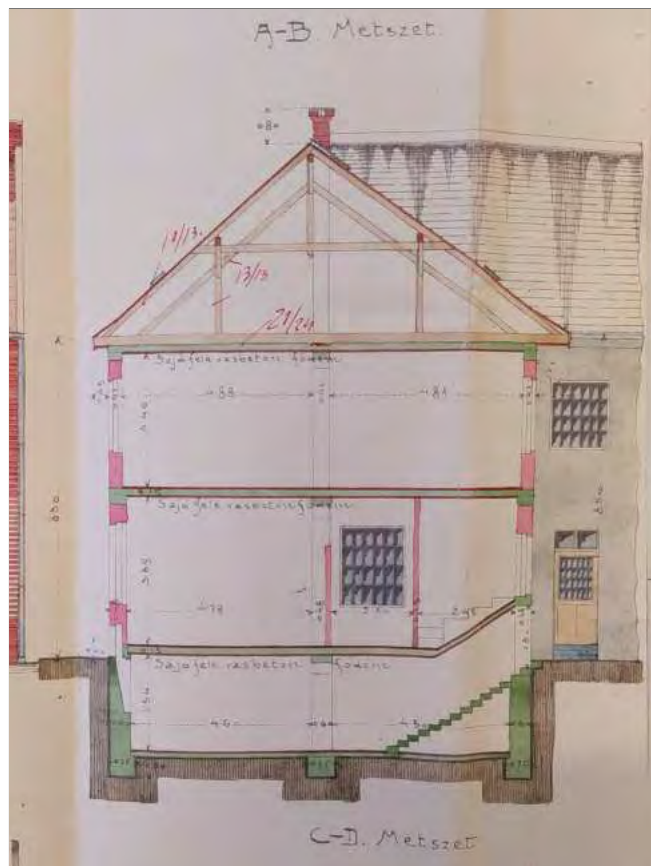
Metszet (módosított terv, 1935.)
