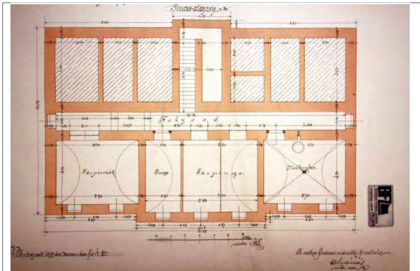
Pince alaprajza
