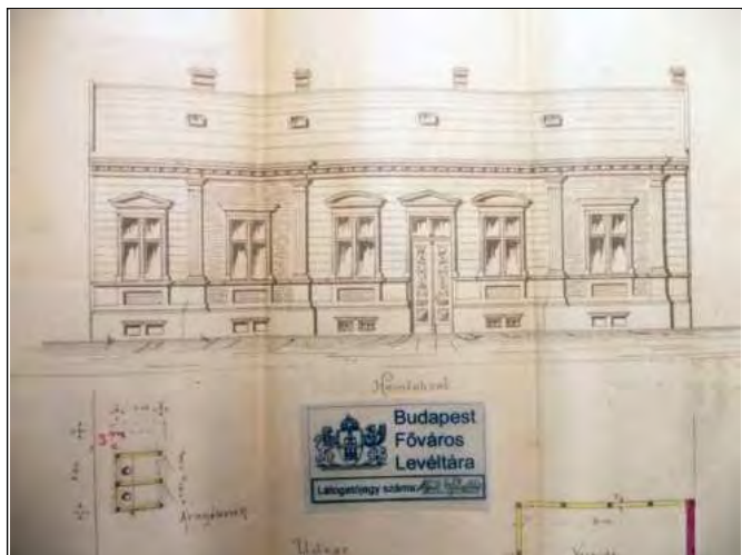
Homlokzati rajz
