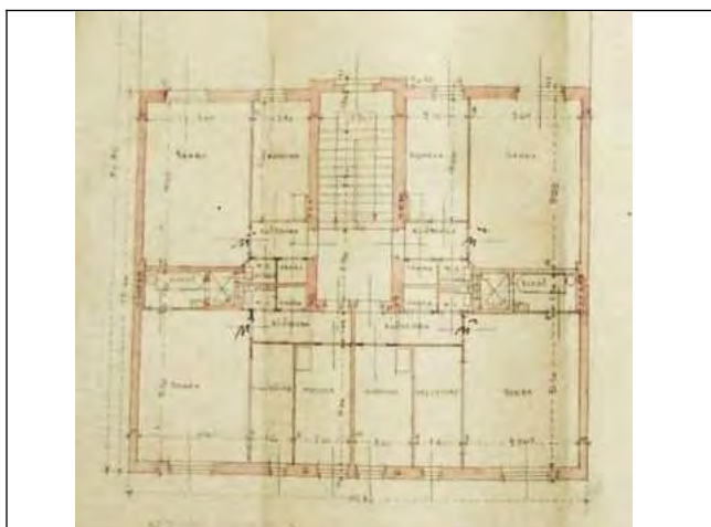
Második emeleti alaprajz
