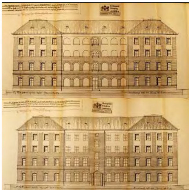
A legénységi lakóházak egyikének homlokzattervei emeletráépítéssel felső: belső tér felé néző homlokzat, alsó: istállók felé néző homlokzat (1924.)
