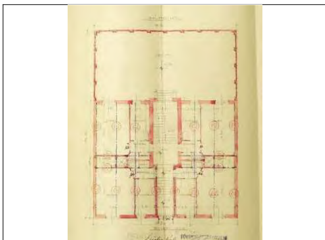
Földszinti alaprajz
