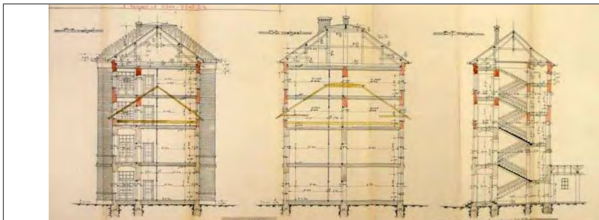
A legénységi lakóházak egyikének metszetrajzai (1924.)
