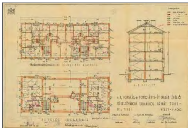
Földszinti, alagsori alaprajz és metszet
