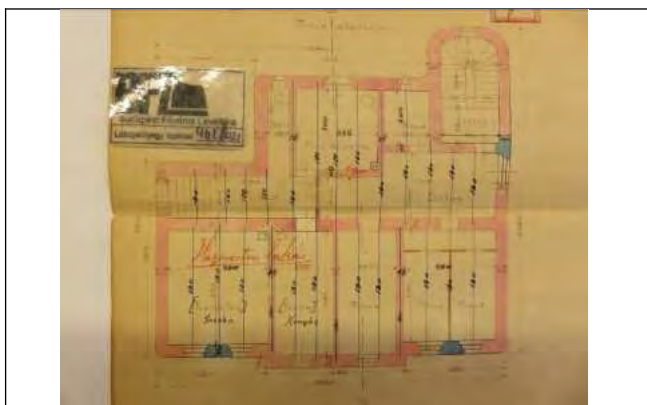
Pince alaprajza
