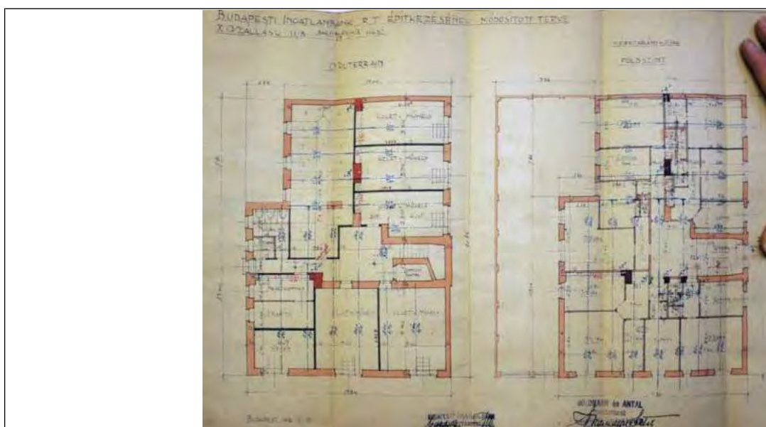
Szuterén és földszinti alaprajz
