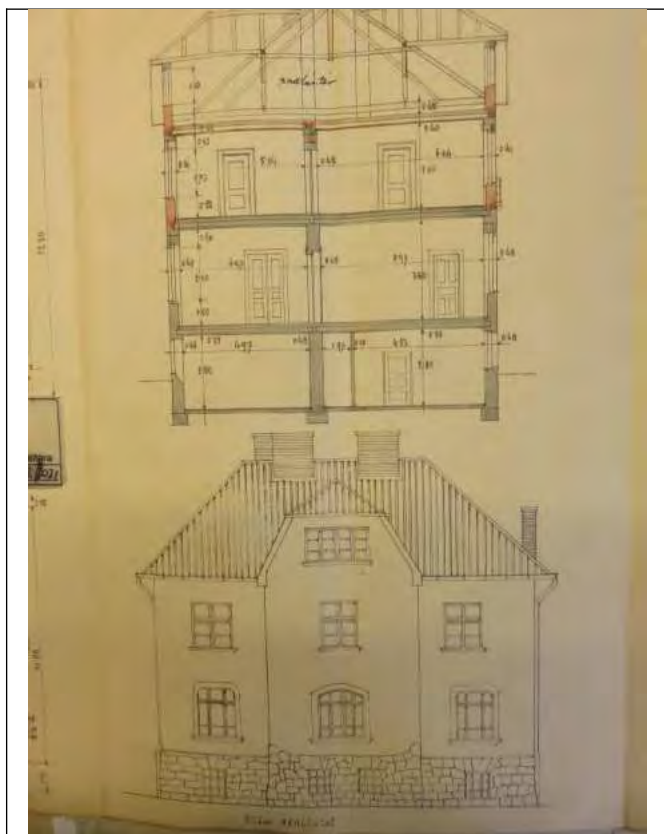
Az emelet-ráépítési terv: metszet és utcai homlokzat
