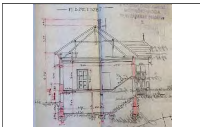
Metszet
