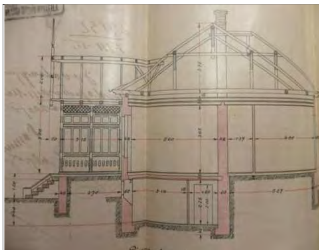
Metszet
