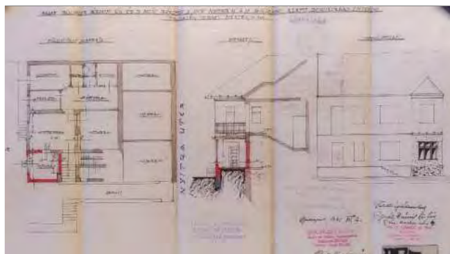
Toldalék terve (1928)
