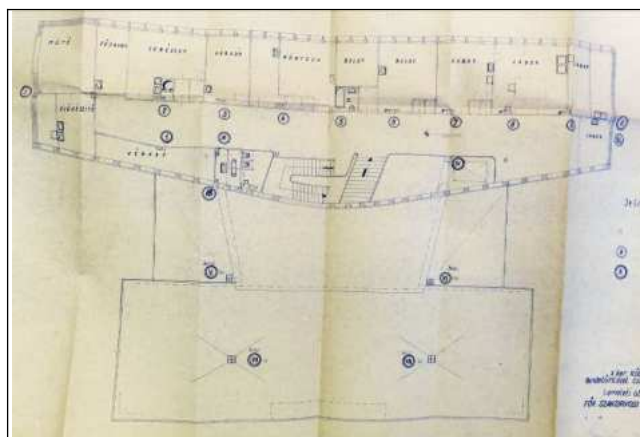
Első emeleti alaprajz (gépészeti korszerűsítés terve – 1966)
