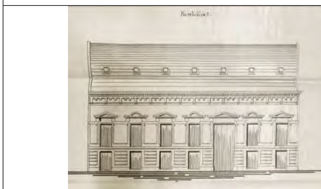
Homlokzat és metszet
