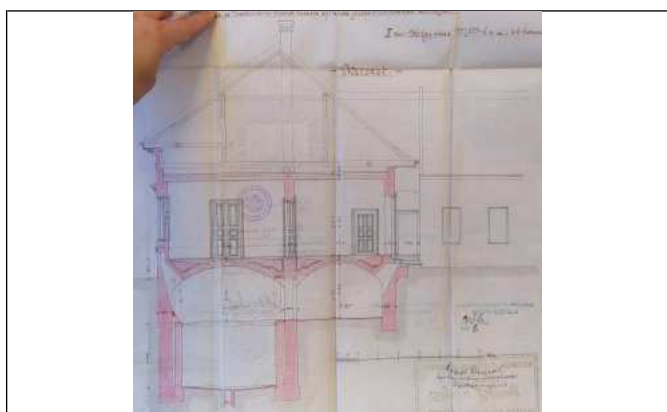
Metszet (1896)
