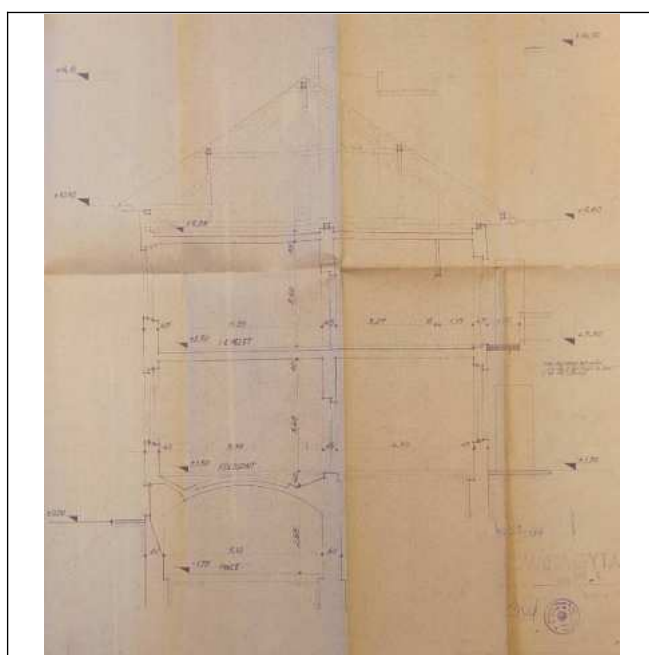
Felújítási terv – Metszet (1964)
