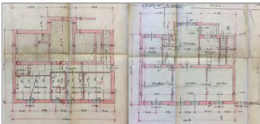
Eredeti tervek – alaprajzok
