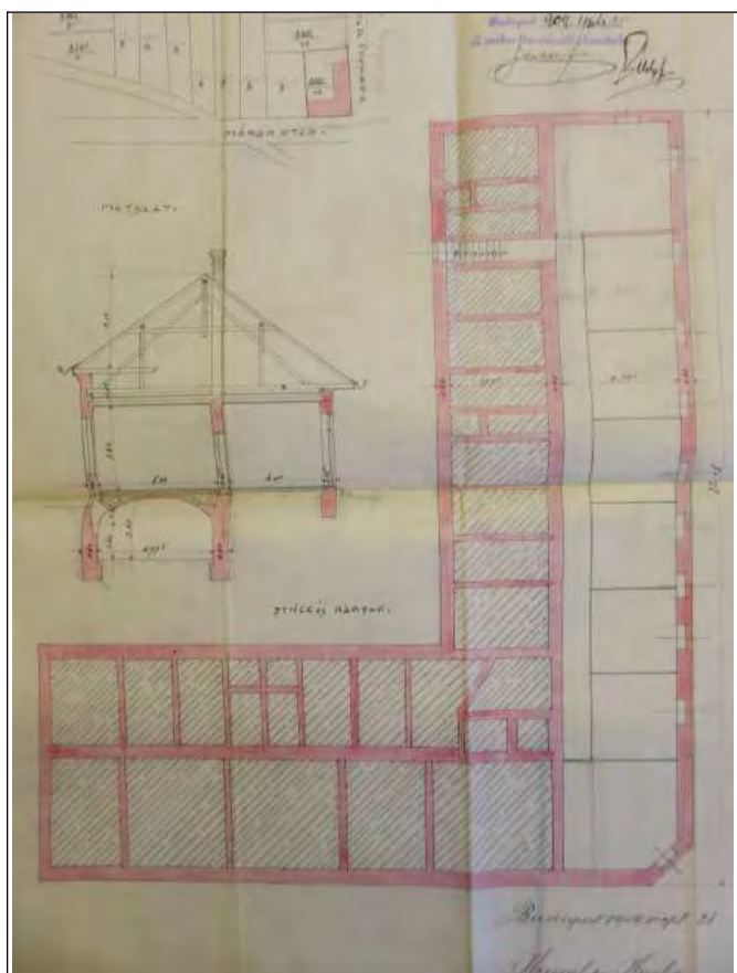
Pincszinti alaprajz és metszet
