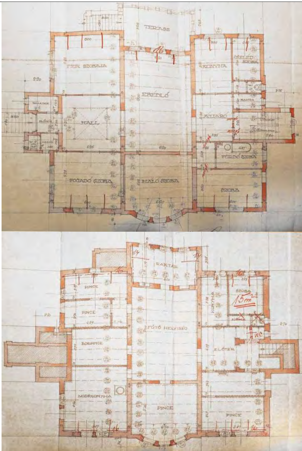
Földszinti és pince alaprajz
