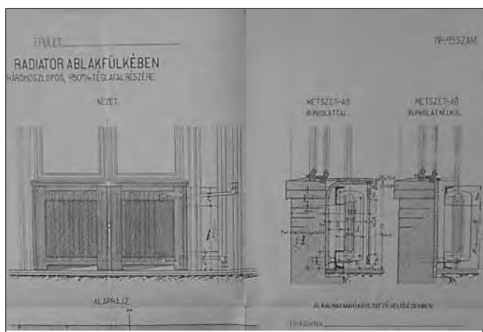
A radiátor elhelyezés részletterve ablakfülkében
