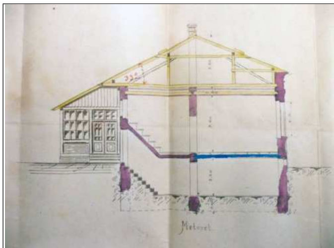
Metszet
