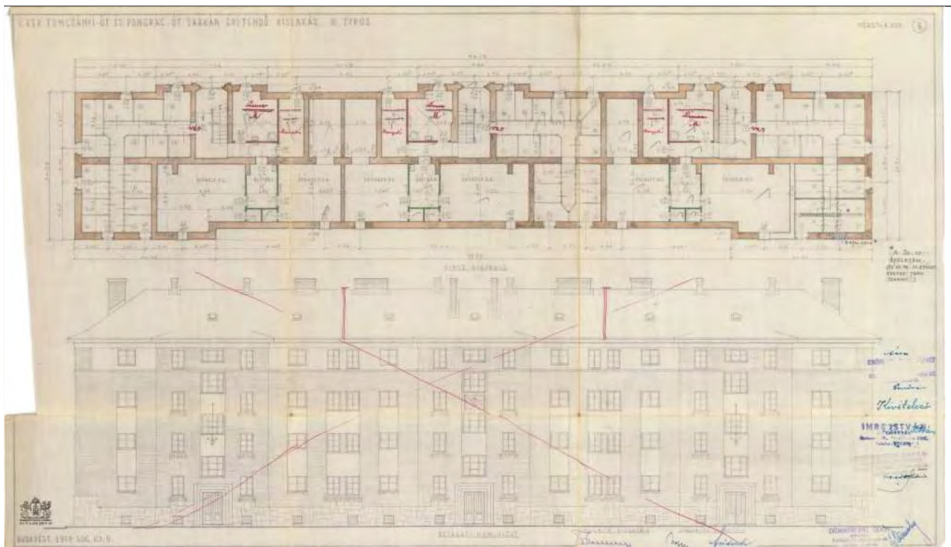
Pince alaprajz és bejárat homlokzat
