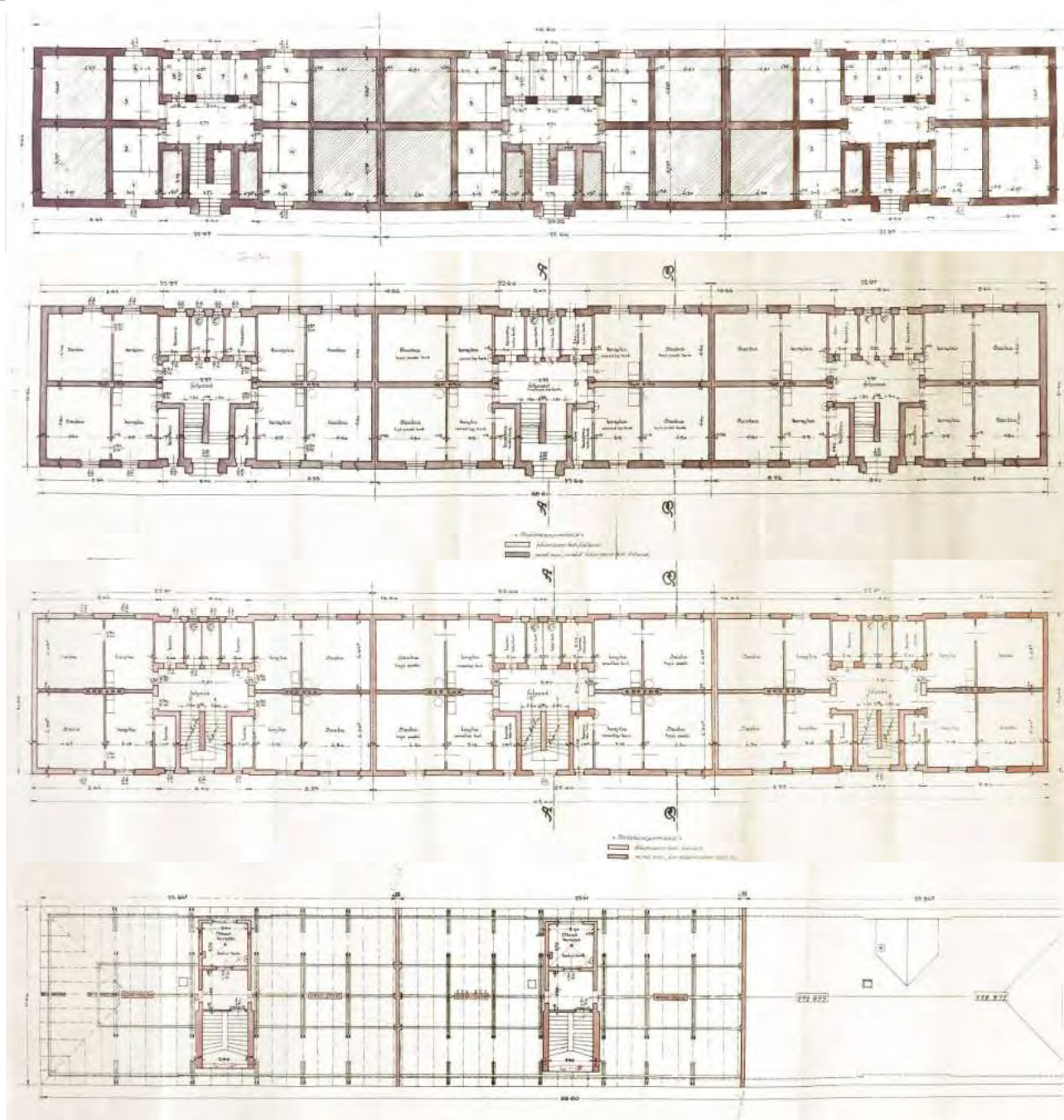
Alaprajzok: pince, földszint, emelet, padlás (fentől lefelé)
