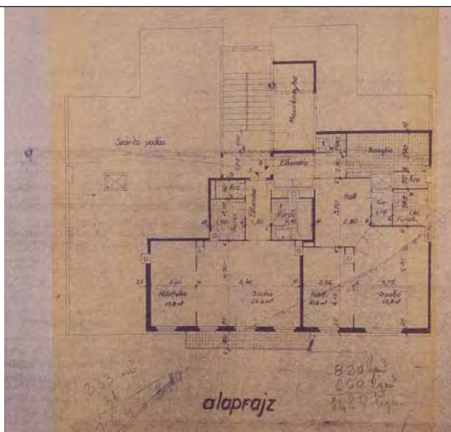
Utólagos tetőemelet alaprajza (1956)
