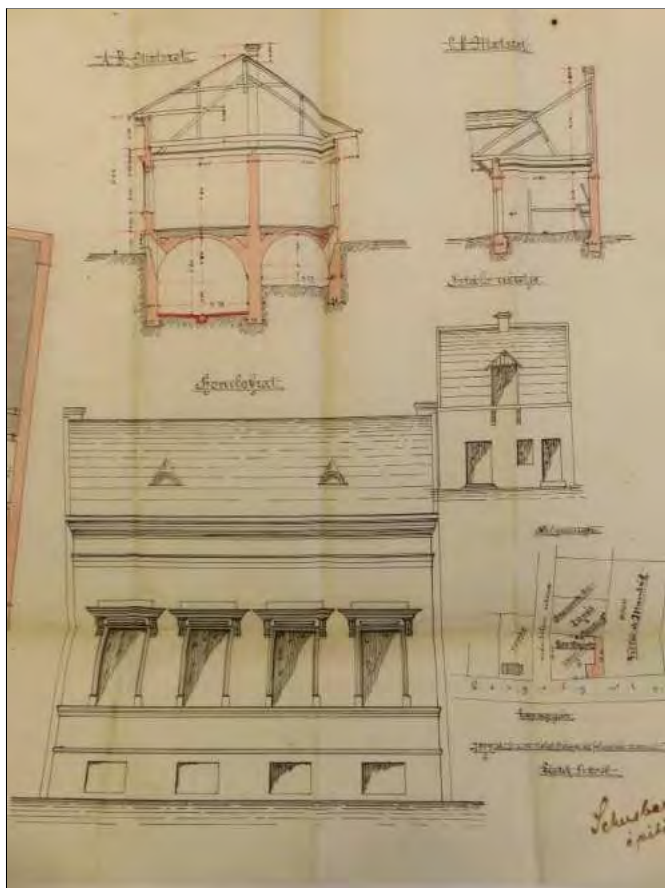
Metszet, homlokzat és helyszínrajz
