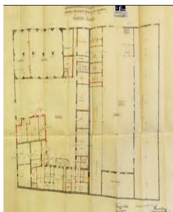
Toldalék és átalakítás alaprajza (1919)
