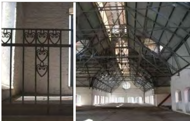
Korlátdíszítés és a csarnok acélszerkezete
