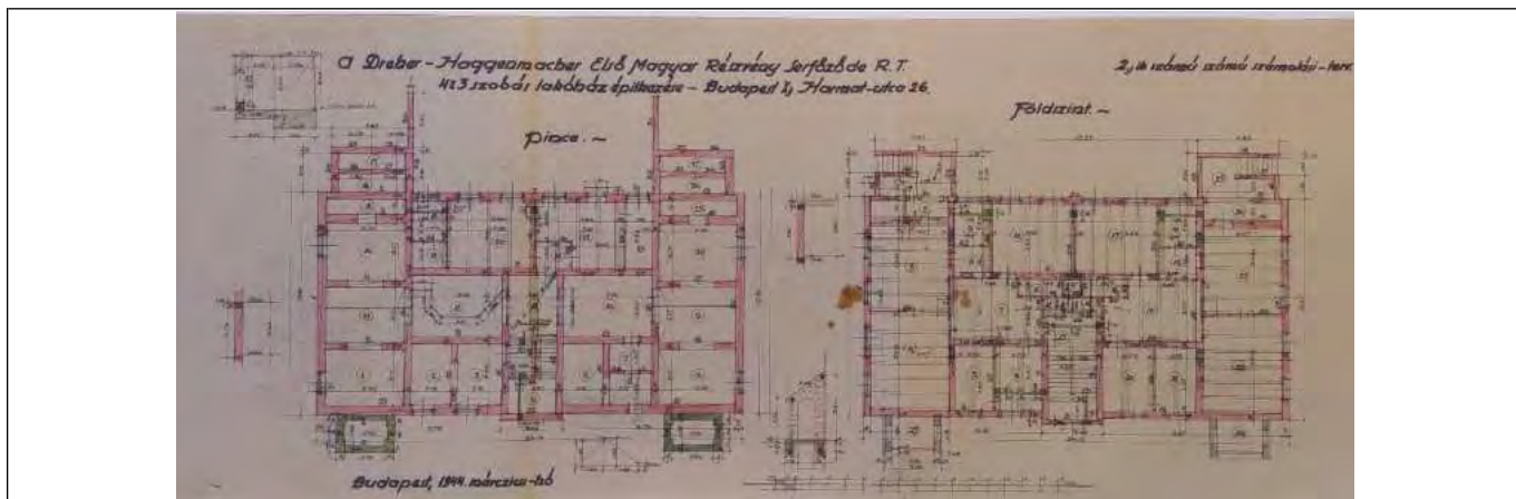
1944-es bővítési terv: alaprajzok
