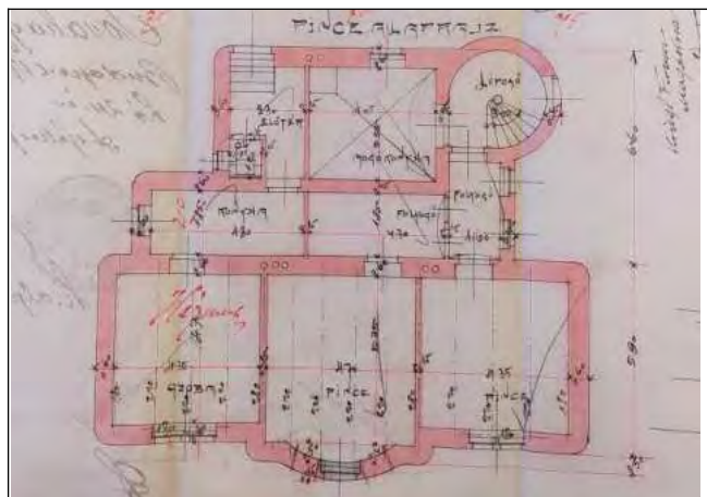
Pincszinti alaprajz
