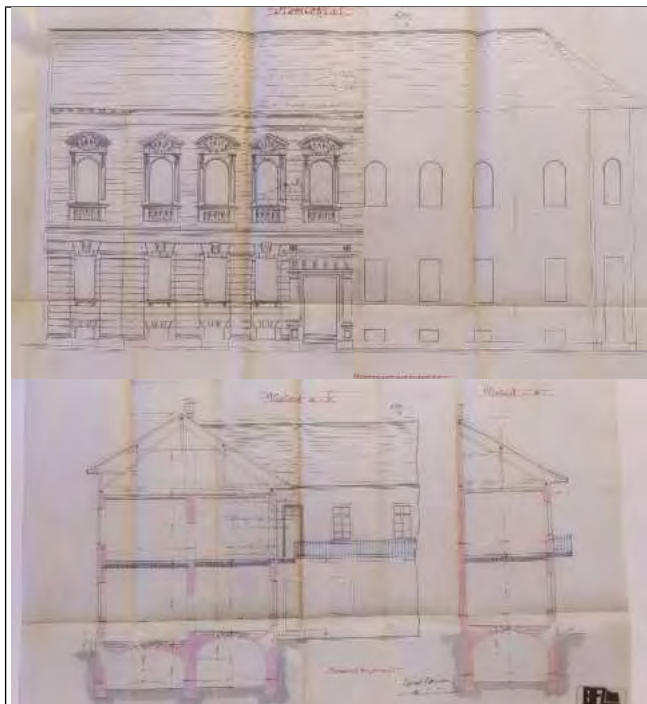
Homlokzat és metszet (1896)
