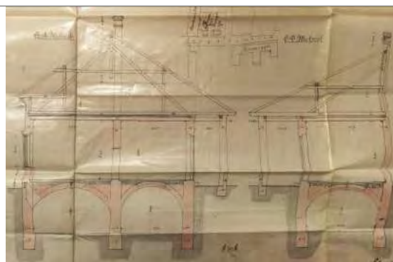
Homlokzat és metszet - Schüsbeck Pál és társa építőmesterek
