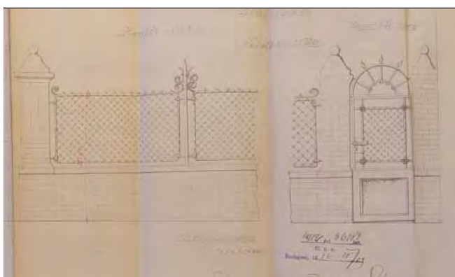
Kerítés terve (1912)
