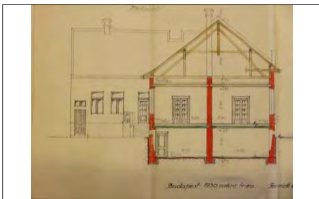
Metszet
