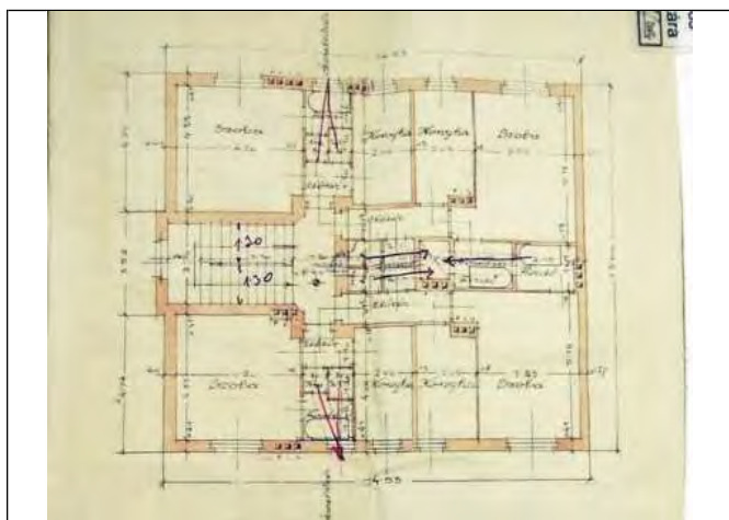
Első emelet alaprajz
