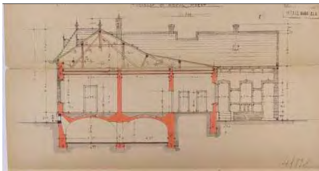
Metszet
