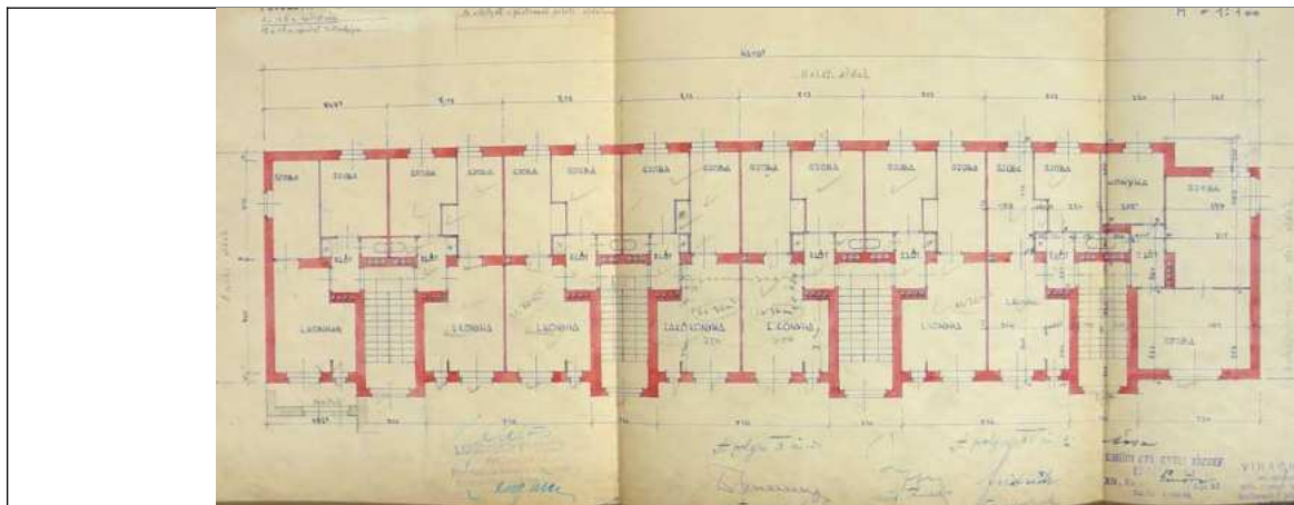
Emeleti alaprajz
