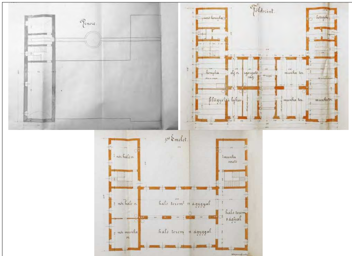
Az eredeti épület tervei: pince, földszint, emelet (balról jobbra) - 1883.
