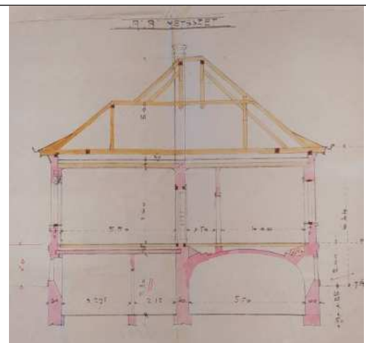
Metszet
