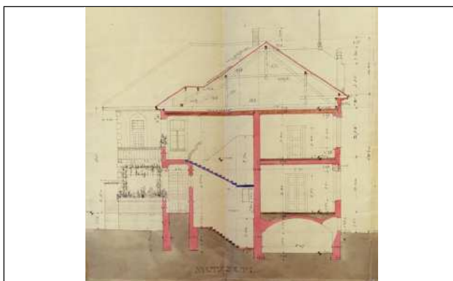
Metszet
