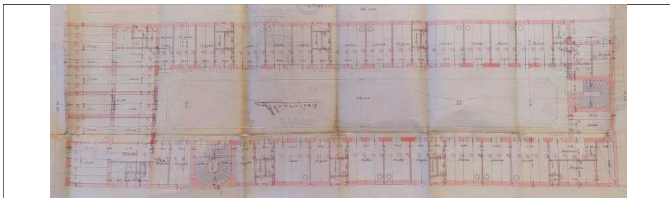
Földszinti alaprajz
