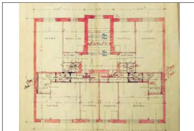
Második emelet alaprajz
