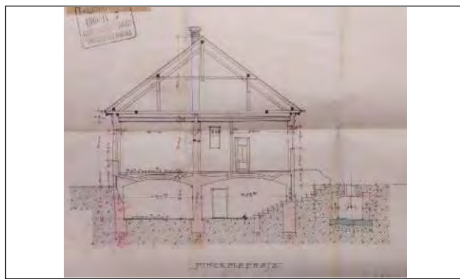
Lakóház metszete
