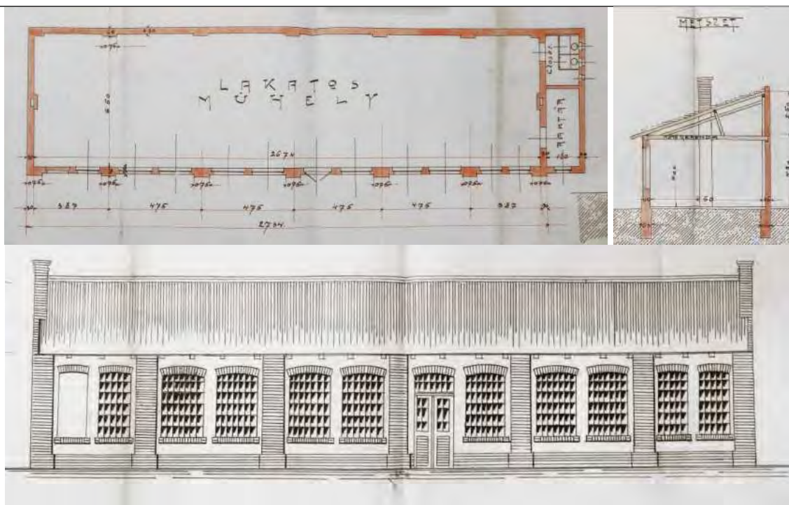
Lakatosműhely alaprajza, metszete és homlokzata
