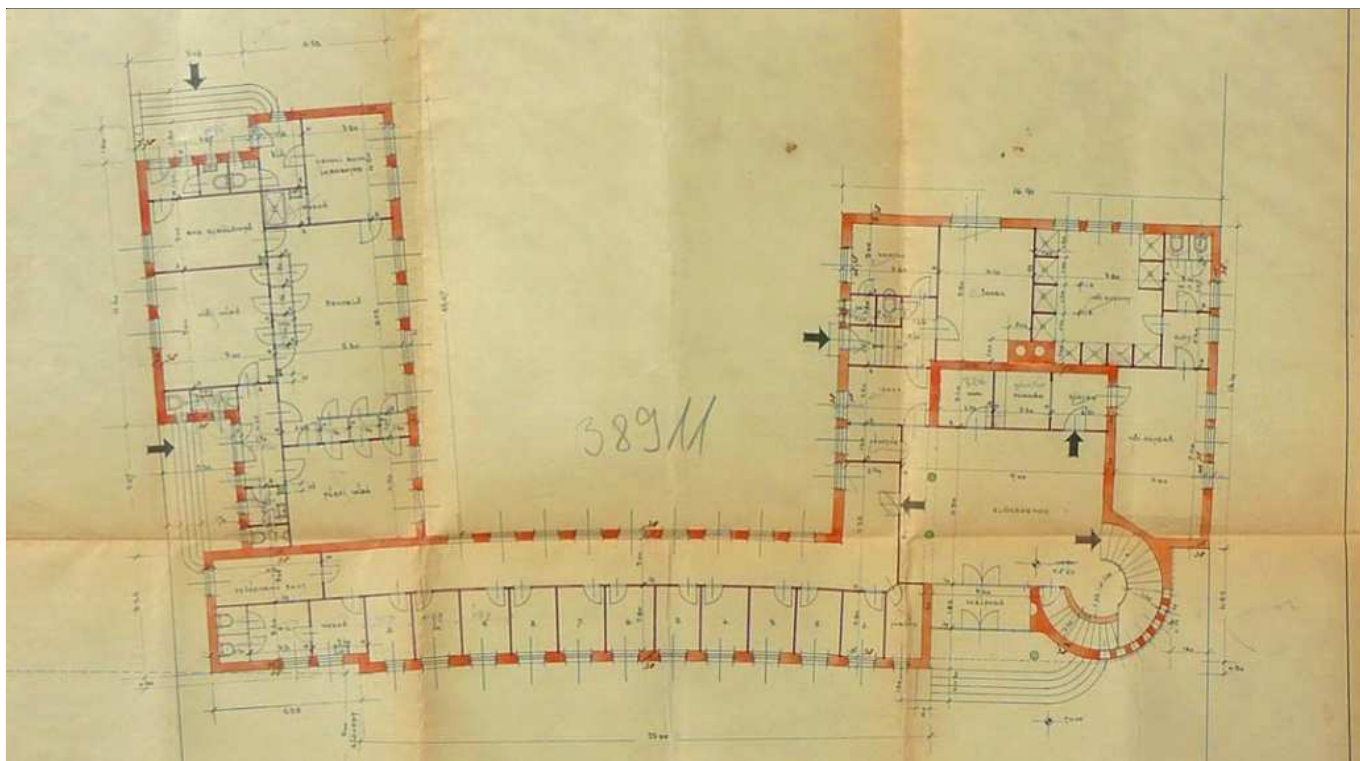
Földszinti alaprajz
