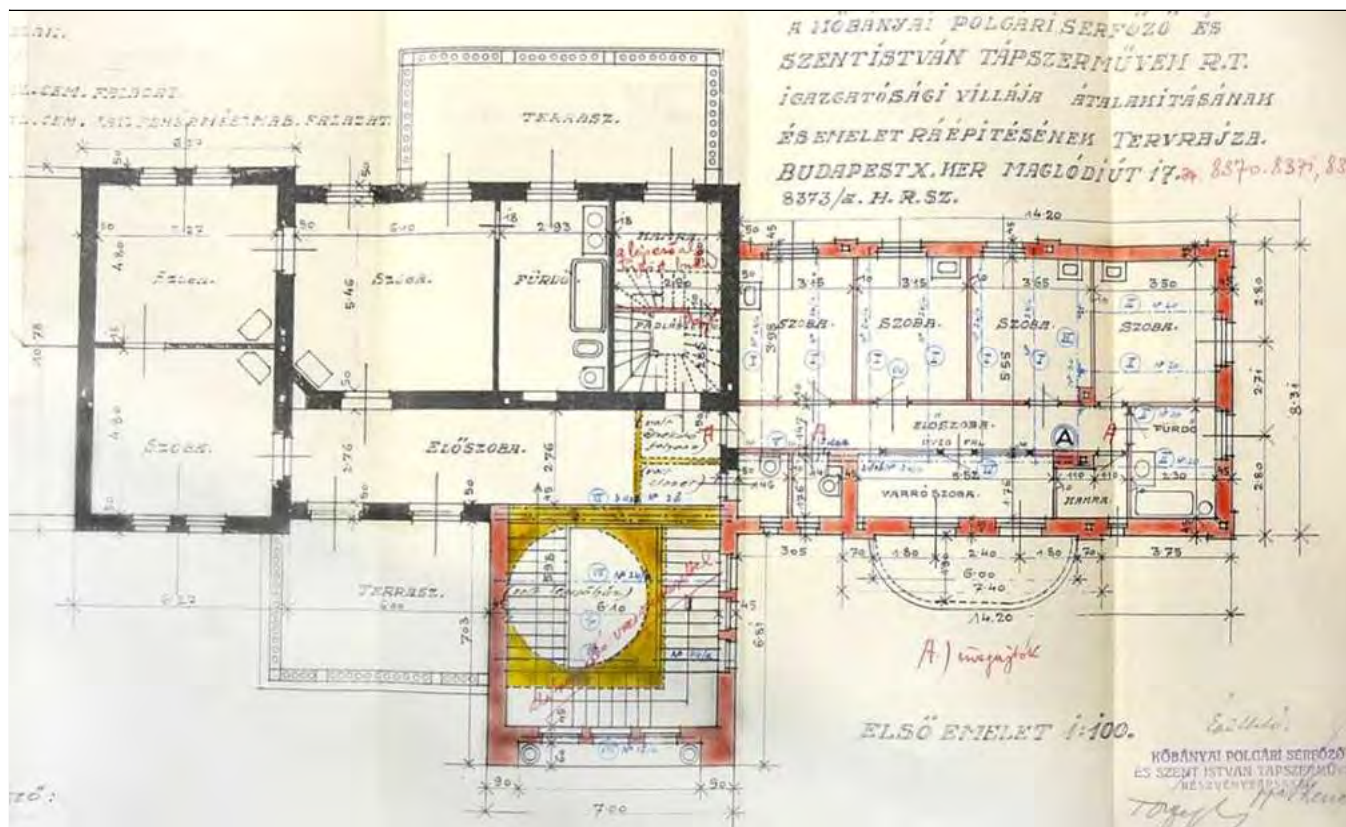
1924. Vidor Emil átalakítási terve
