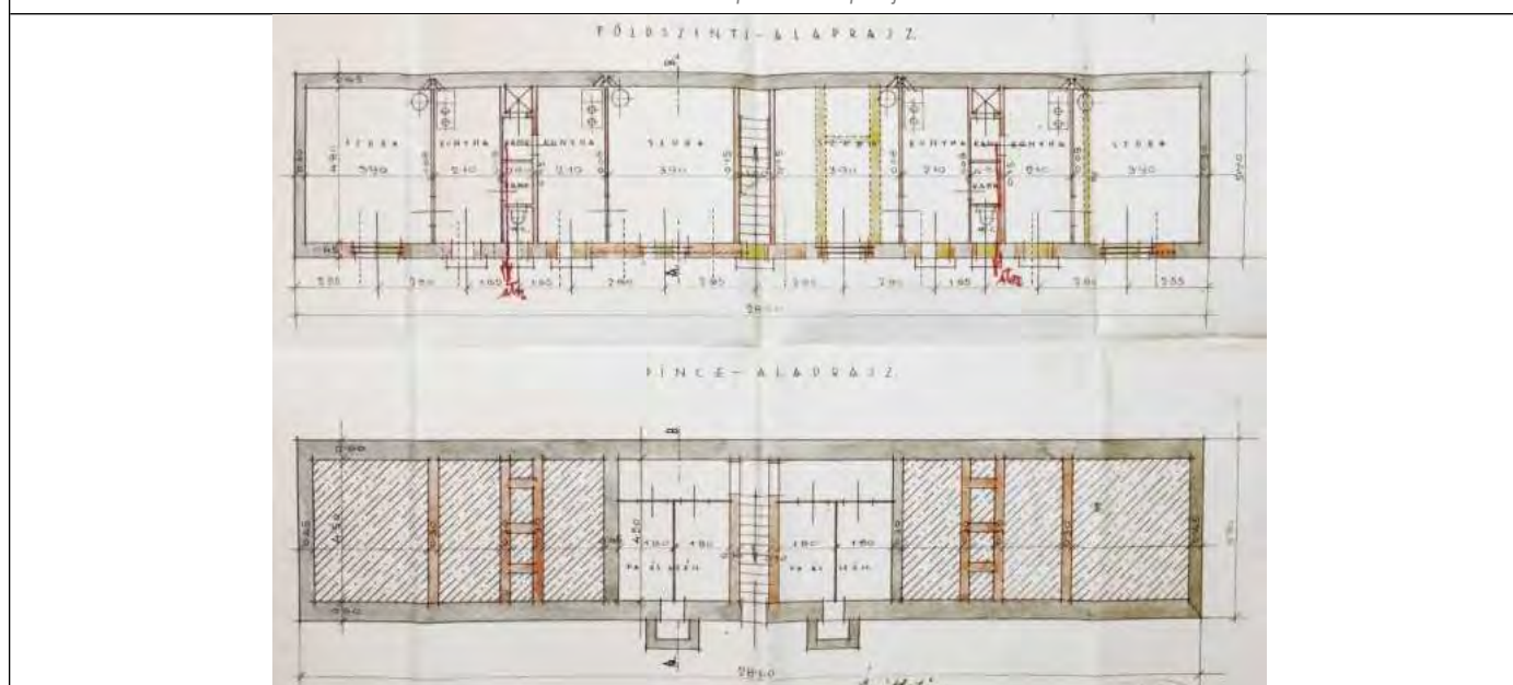
A melléképület átalakítási alaprajza (1937)
