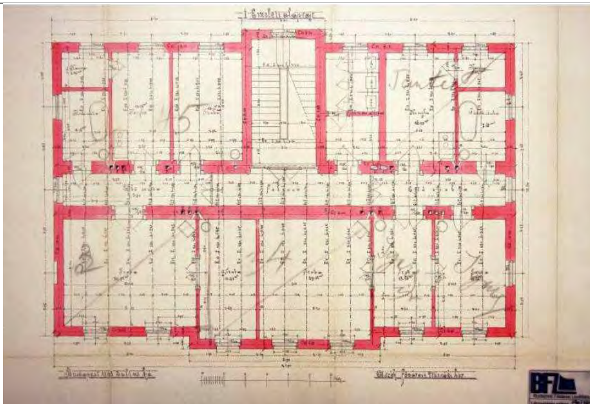
Emeleti alaprajz
