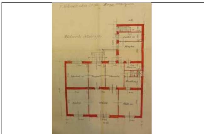
Földszinti alaprajz
