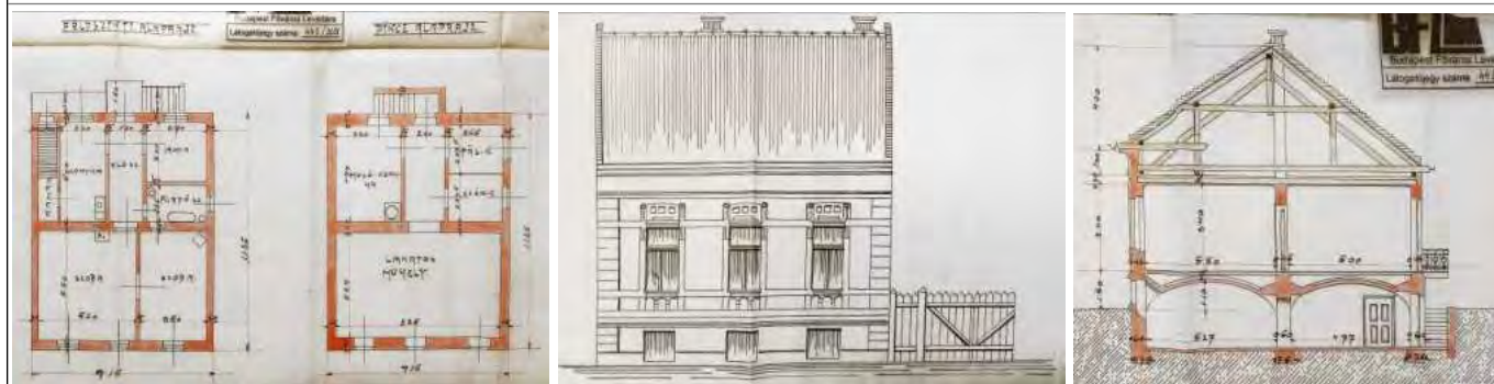
Lakóépület földszinti és pince alaprajza, illetve homlokzata és metszete 1908.
