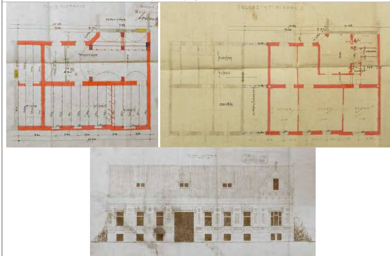
Lakóépület átalakításának pince és földszint alaprajza, illetve az átalakítás homlokzati terve- 1911.
