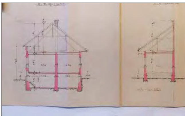
Metszet
