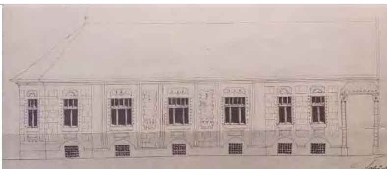
Homlokzatok
