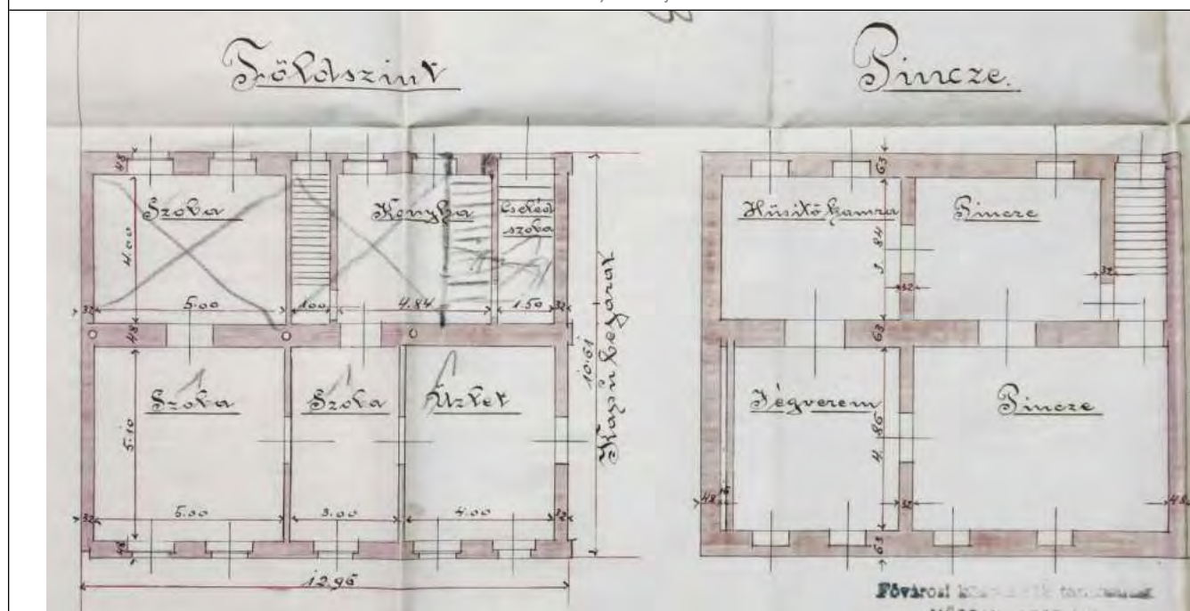
Lakóépület földszinti és pince alaprajza
