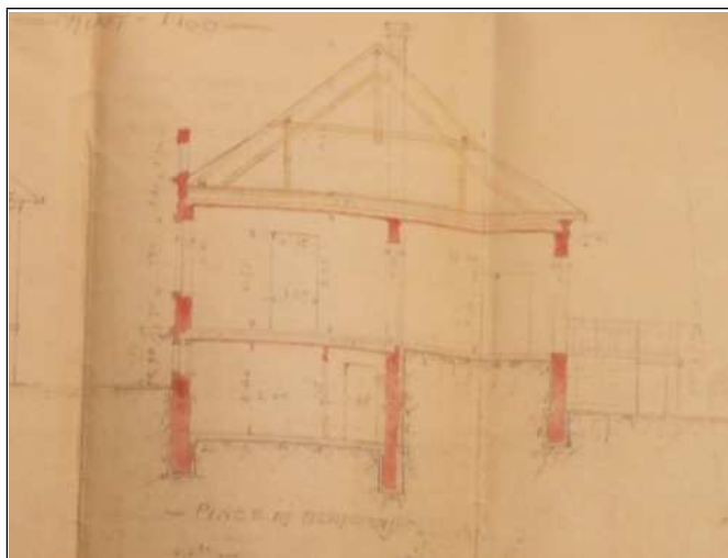
Metszet
