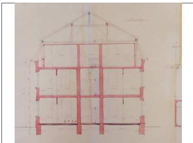
Metszet
