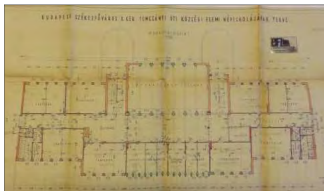
Magasföldszinti alaprajz
