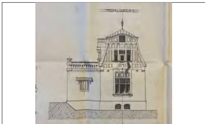
Homlokzat
