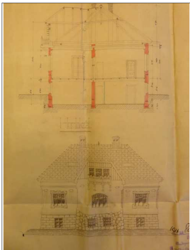
Az eredeti tervek: metszet és homlokzat
