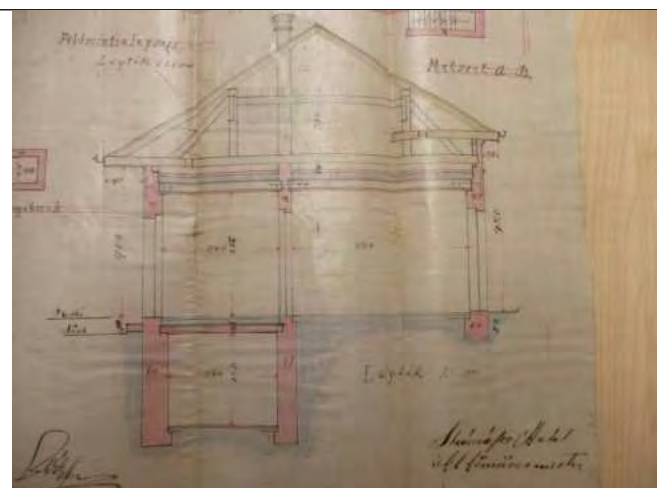
Metszet
