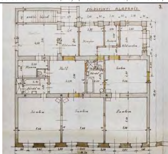
Átalakítási földszinti alaprajz (Sorg Antal építőmester) 1939.
