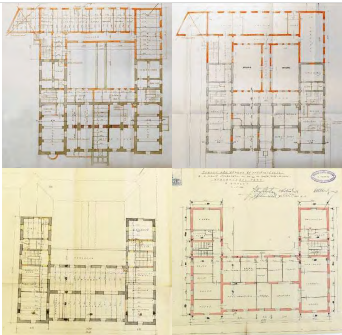
Átalakítás és bővítés alaprajzai: alagsor, földszint, 1. emelet, 2. emelet (balról jobbra) 1928.
