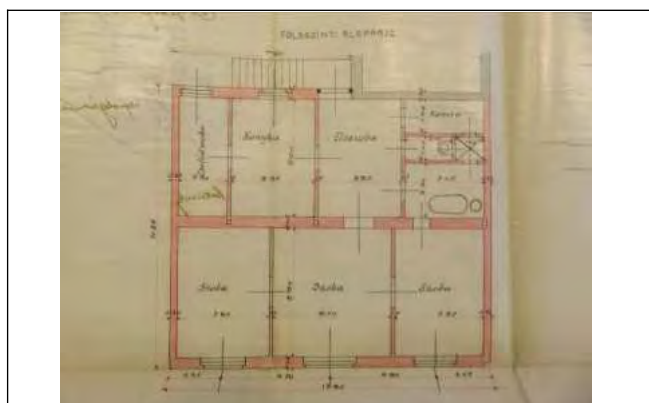
Földszinti alaprajz
