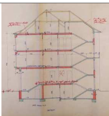
Tetőemelet ráépítés előtti metszet terve (1942)
