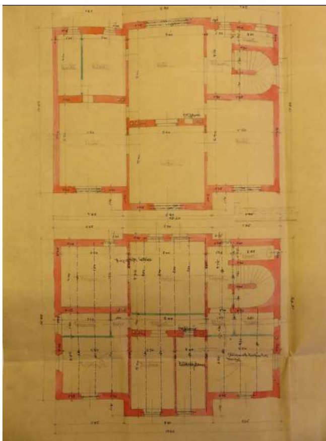
Az eredeti tervek: alaprajzok
