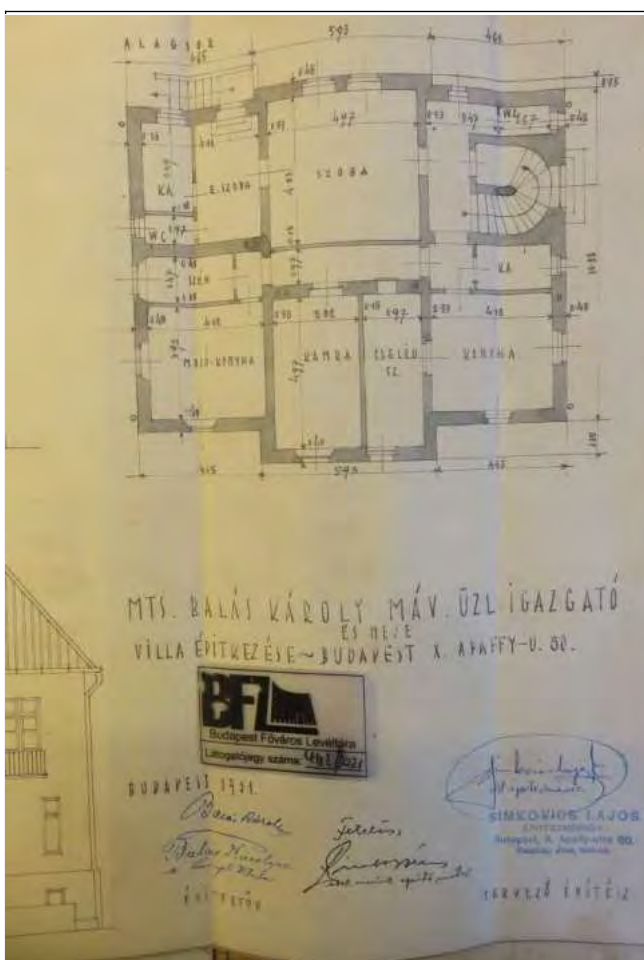
Meglévő alagsori alaprajz az emelet-ráépítési terven
