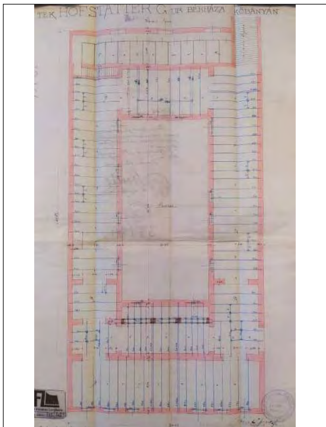
1894-es bérház terve – pince alaprajz
