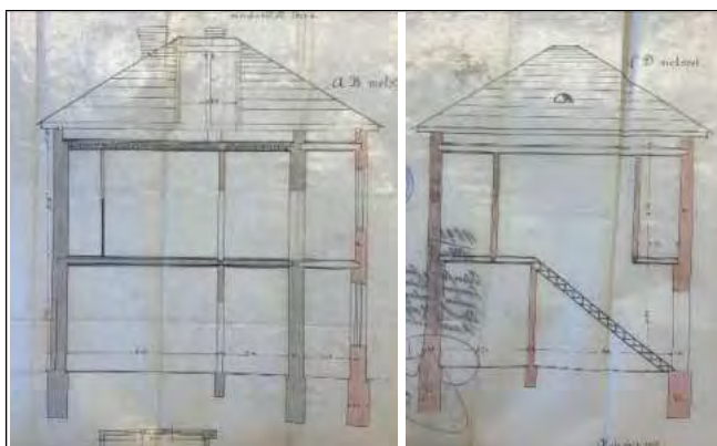
Metszetek (toldalékterv, 1899)
