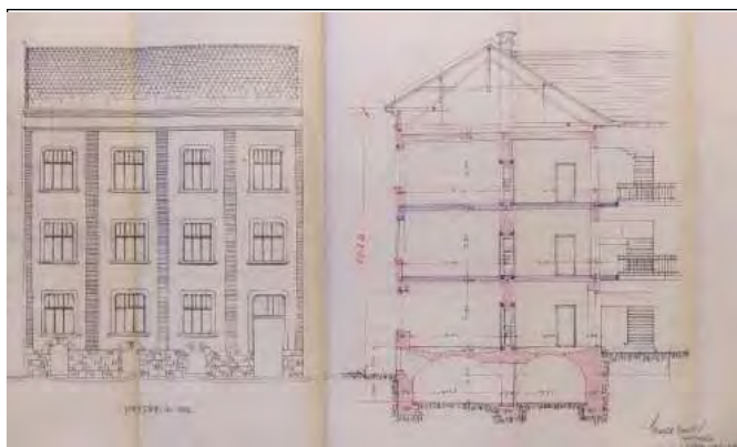
Eredeti terv – homlokzat, metszet (1914)
