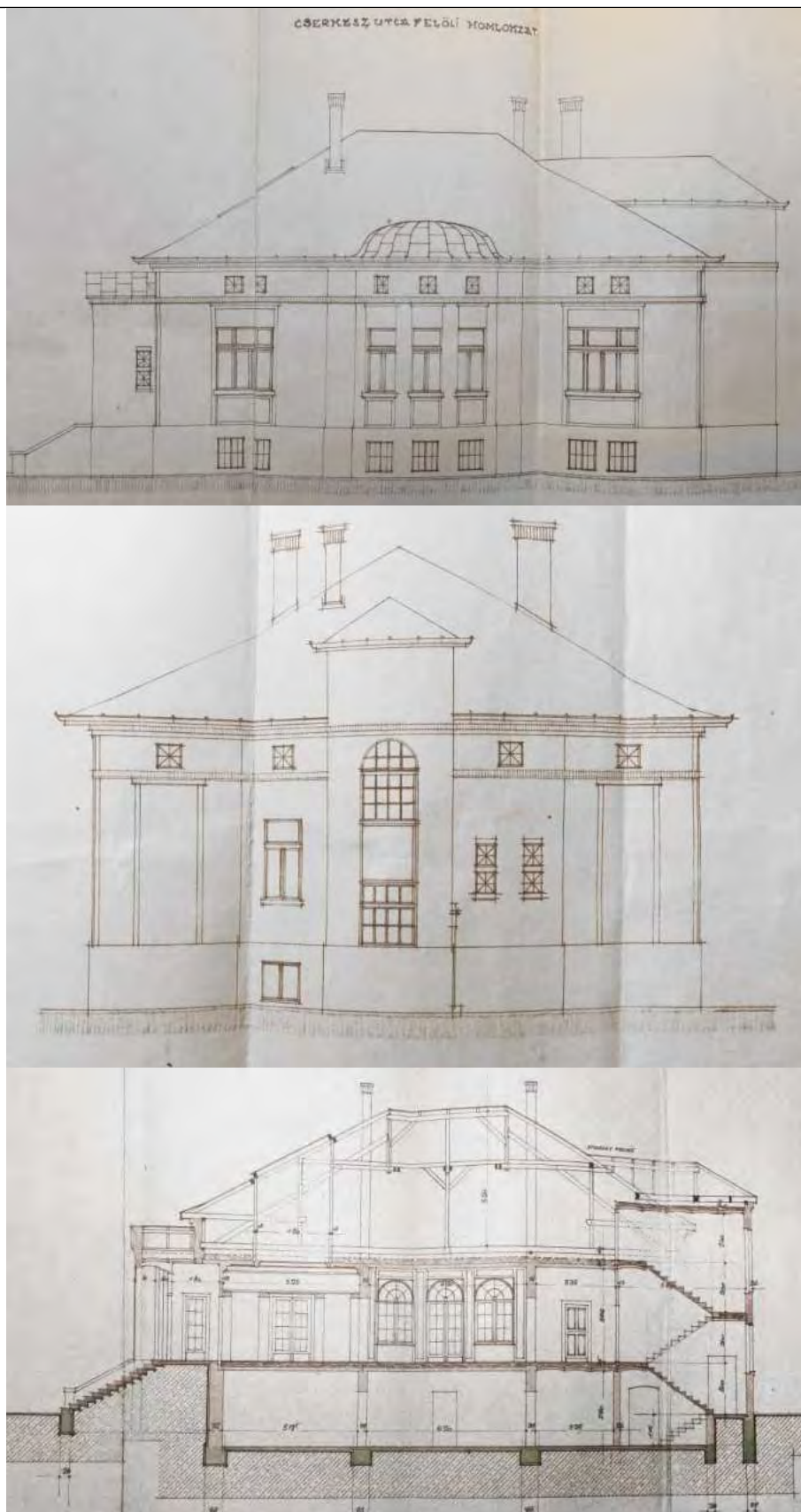
Homlokzatok és metszet
