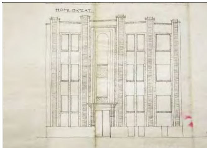
Homlokzati rajz
