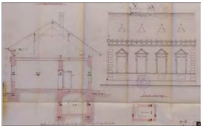
Metszet és homlokzat
