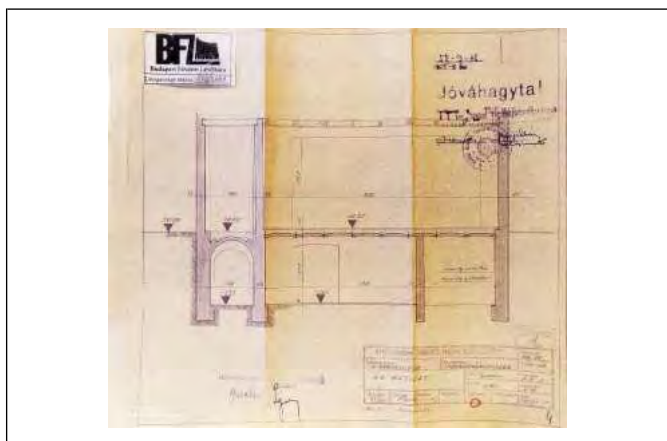
Homlokzati terv (1955)
