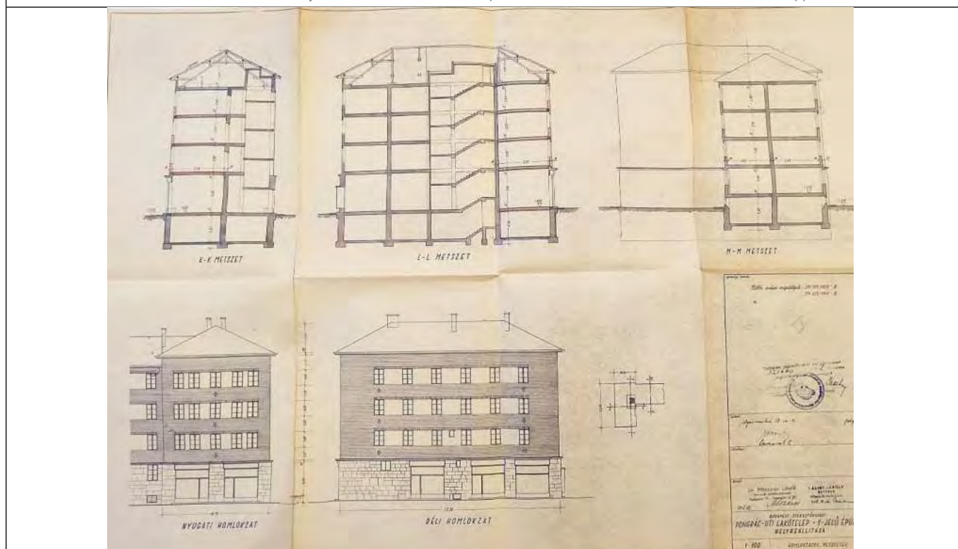
A háborús károk kijavítására készült terv (1948, Dr. Mészáros László, Bálint Károly)
