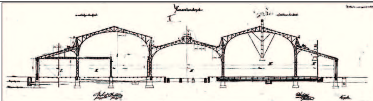
A csarnok korabeli metszete
