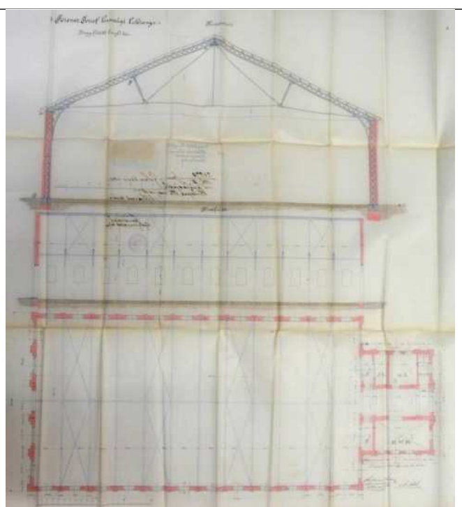
A központi udvartól (felállóhely) délre található nagy fedett lovarda tervei
