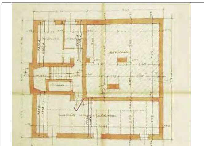
Pincszinti alaprajz
