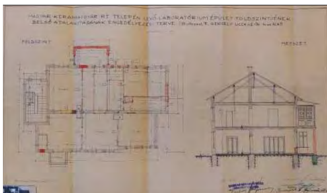
Laboratórium épület földszintjének belső átalakítási terve (1936)
